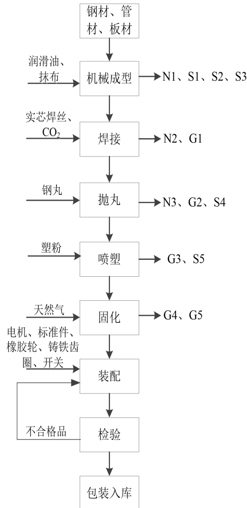
图 2-4 扫雪机生产工艺流程图
