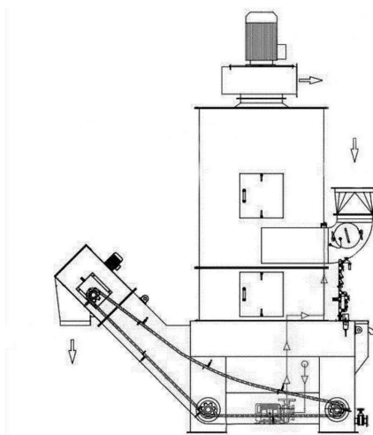
图 4-5 湿式除尘装置结构示意图
