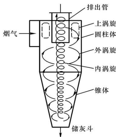
图 4-4 旋风除尘装置结构示意图
