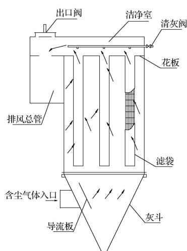
图 4-3 布袋除尘器结构示意图
