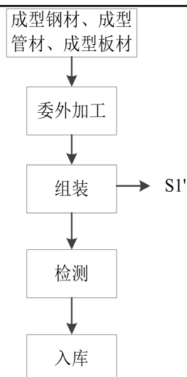
图 2-5 小型搅拌机组装工艺流程图
