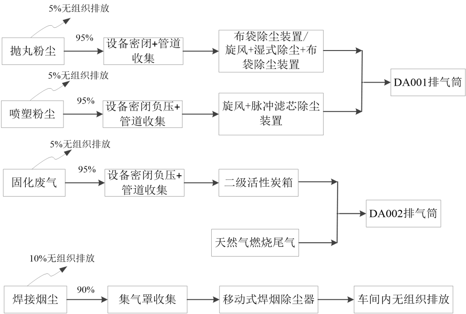
图4-1 废气收集、处理、排放流程图
