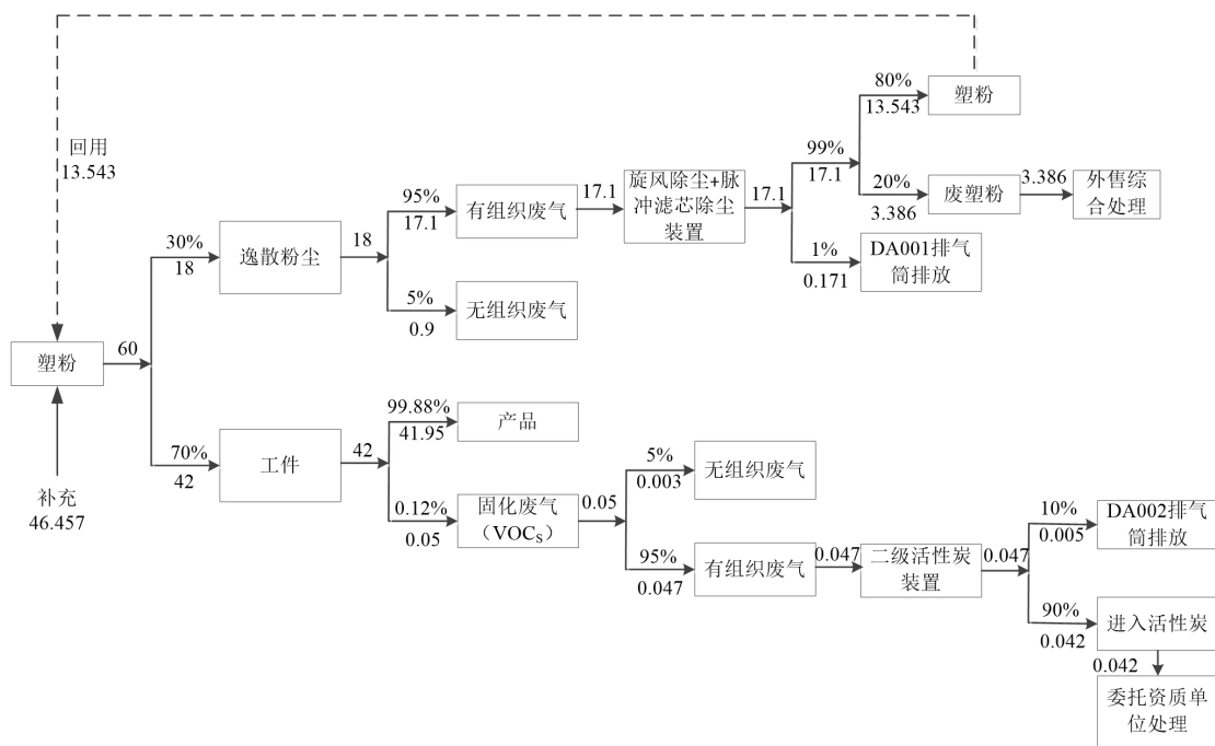
图 2-1 本项目塑粉物料平衡图
