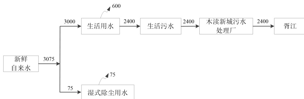
图 2-3 扩建后全厂水平衡图
