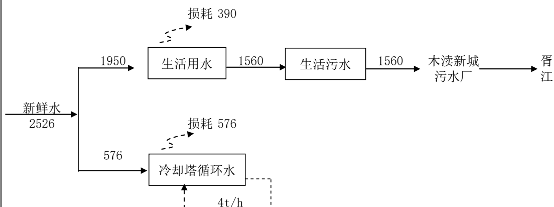
图 2-1 本项目水平衡图 (m³/a)
