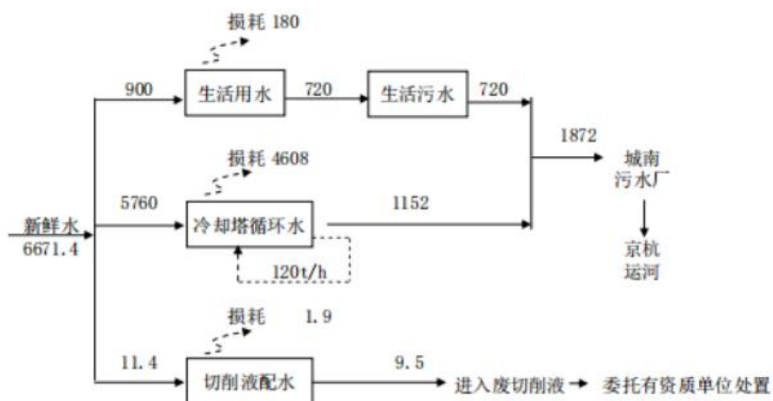
图 2-1 本项目建成后全厂水平衡图 (t/a)
