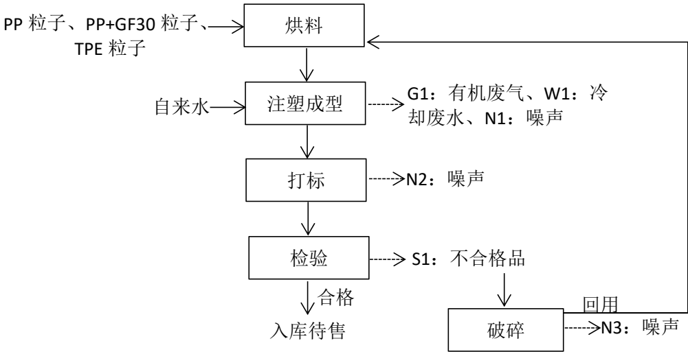
图 2-2 注塑件生产工艺流程
