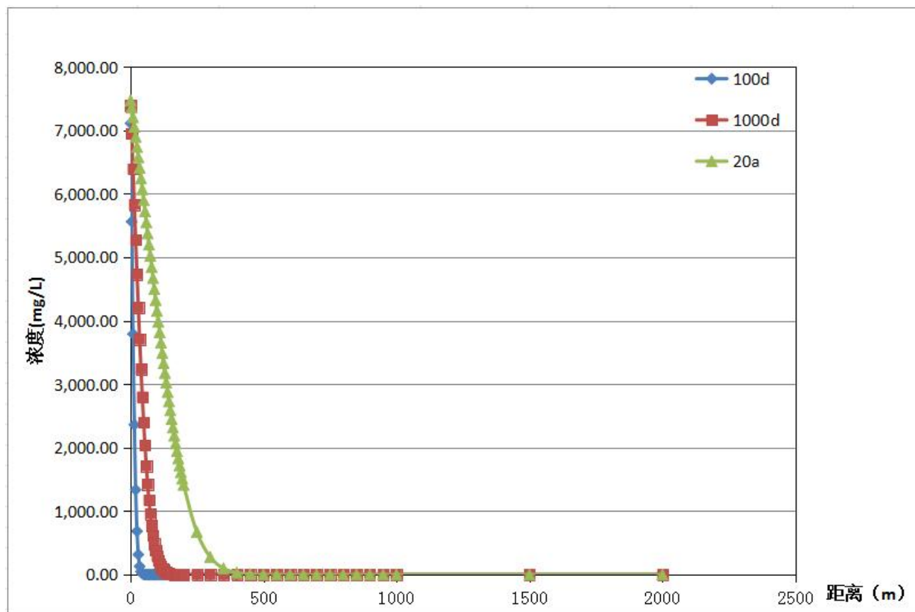
图 7.5-4 污染物 COD Mn 浓度迁移变化预测图
