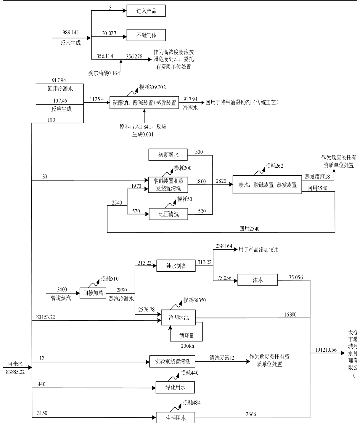
图 4.5-34 本项目建成后全厂水平衡图 (t/a)
