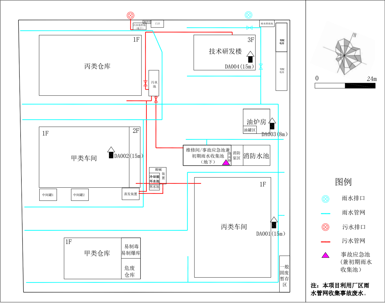
图 8.7-5 厂区雨、污水管网及事故应急池分布图
