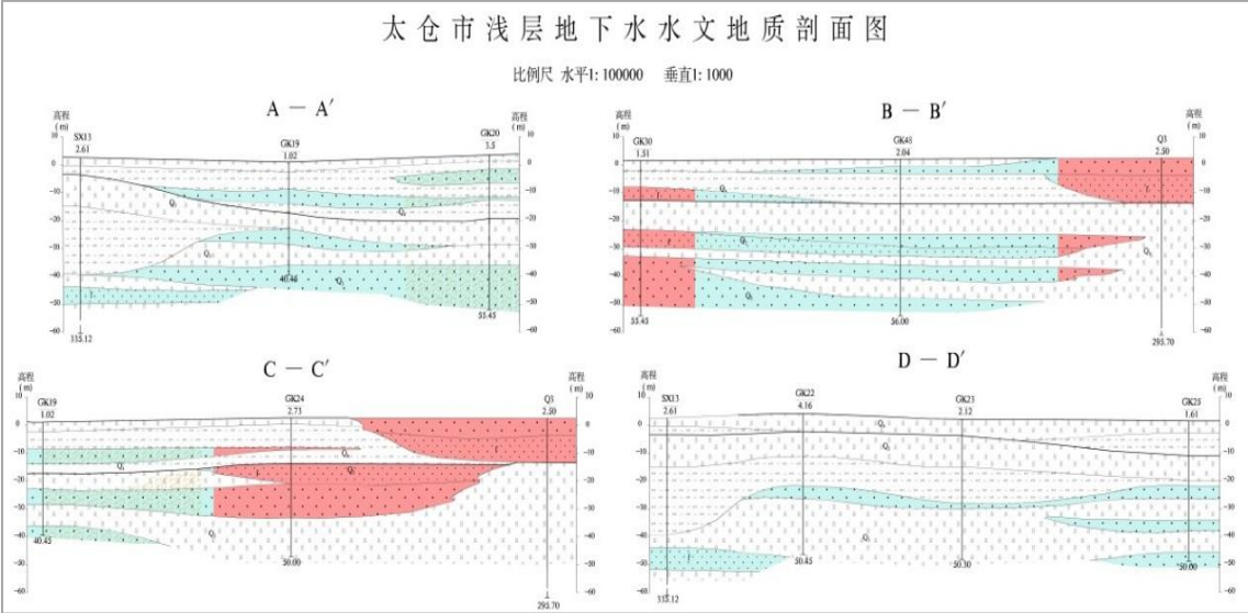
图 7.5-3 区域浅层地下水水文地质剖面图
