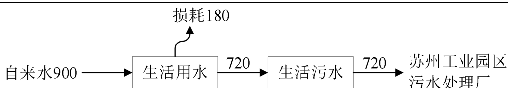
图 2-1 本项目水平衡图 (t/a)
