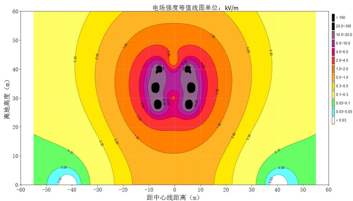
图 3-5 220kV 尚万线新建段架空线路工频电场强度达标等值线图
