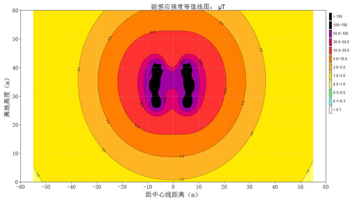
图 3-6 220kV 尚万线新建段架空线路工频磁感应强度达标等值线图
