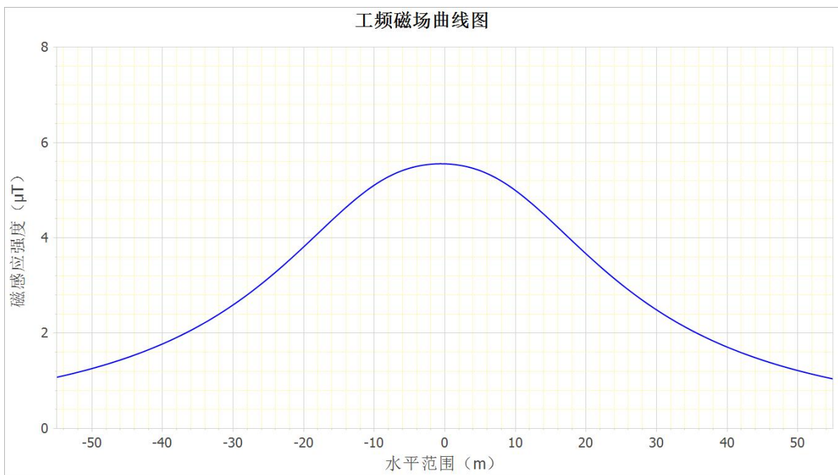
图 3-4 220kV 尚万线恢复架线段架空线路下工频磁场随距离变化趋势图
