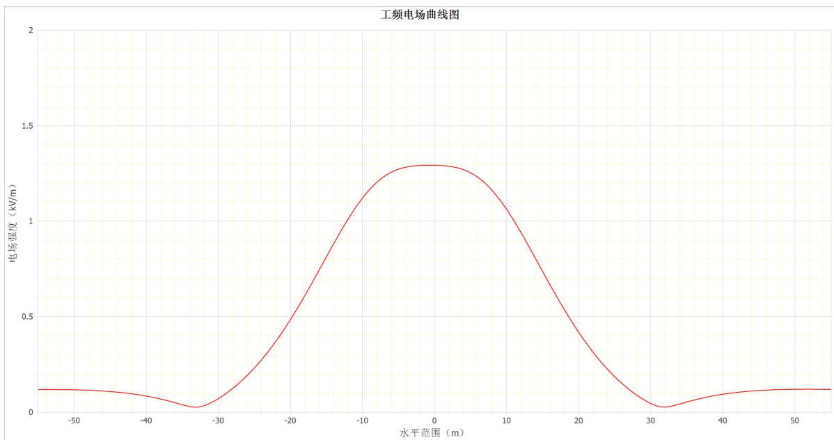
图 3-3 220kV 尚万线恢复架线段架空线路下工频电场随距离变化趋势图
