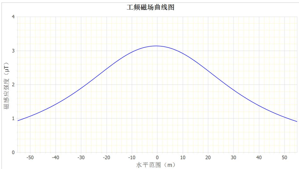
图 3-2 220kV 尚万线新建段架空线路下工频磁场随距离变化趋势图
