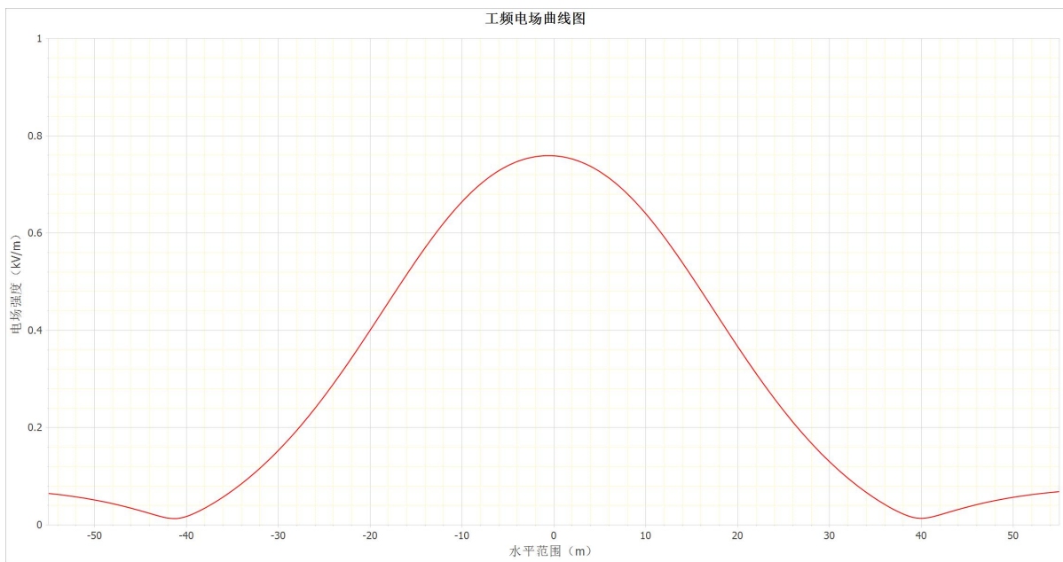
图 3-1 220kV 尚万线新建段架空线路下工频电场随距离变化趋势图
