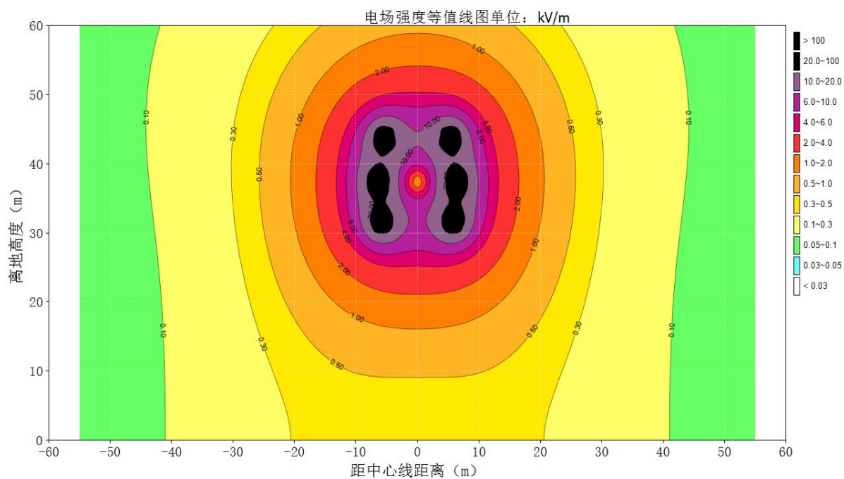
图 3-5 220kV 熟剑线新建段架空线路工频电场强度达标等值线图
