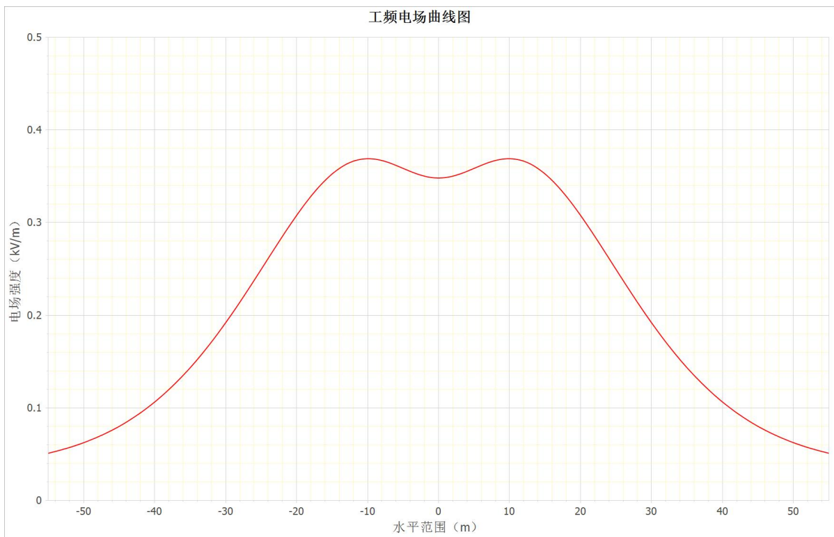
图 3-1 220kV 熟剑线新建段架空线路下工频电场随距离变化趋势图
