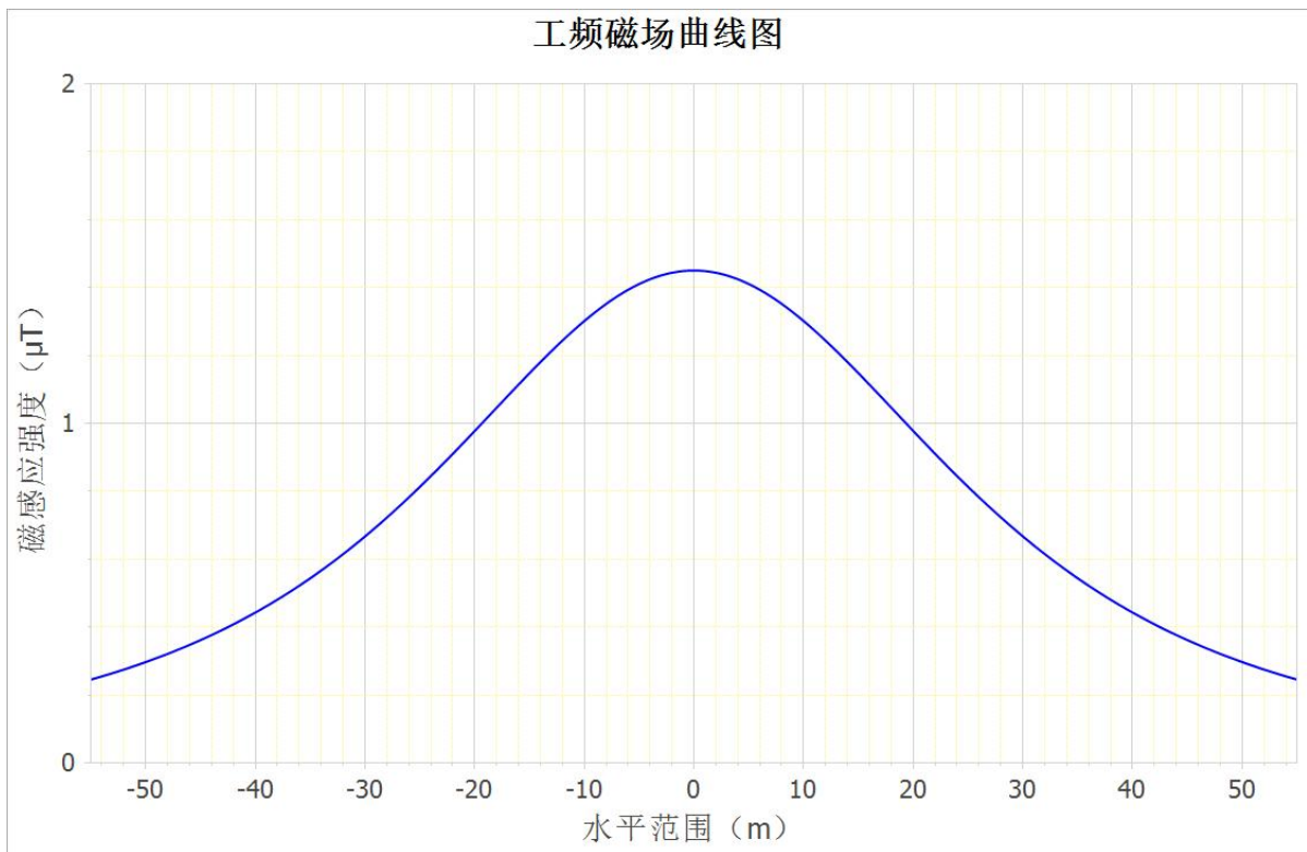
图 3-2 220kV 熟剑线新建段架空线路下工频磁场随距离变化趋势图
