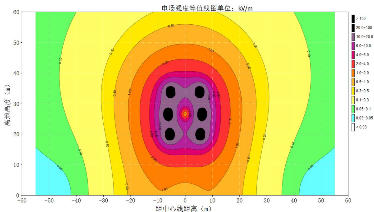
图 3-7 220kV 熟剑线恢复架线段架空线路工频电场强度达标等值线图
