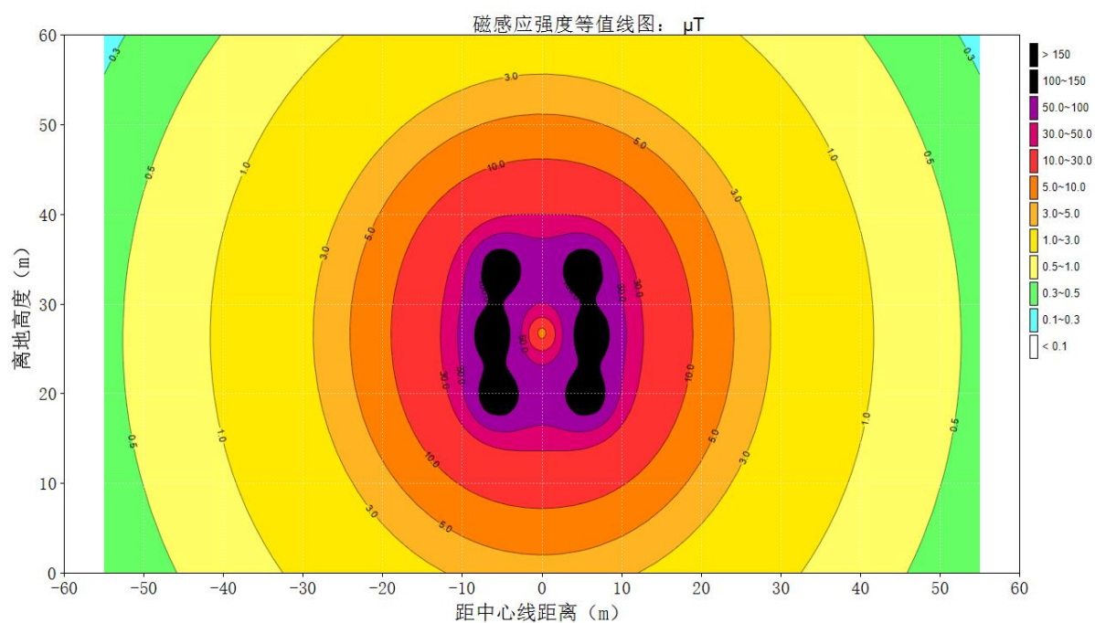
图 3-8 220kV 熟剑线恢复架线段架空线路工频磁感应强度达标等值线图
