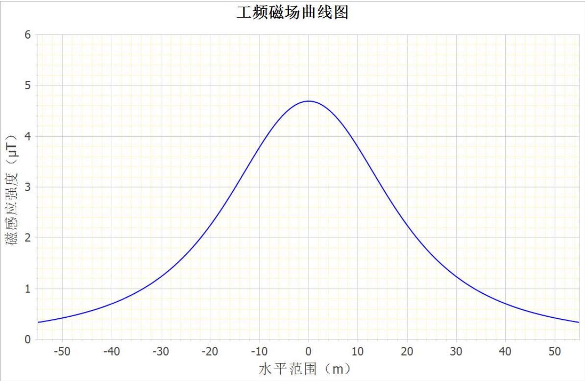
图 3-4 220kV 熟剑线恢复架线段架空线路下工频磁场随距离变化趋势图
