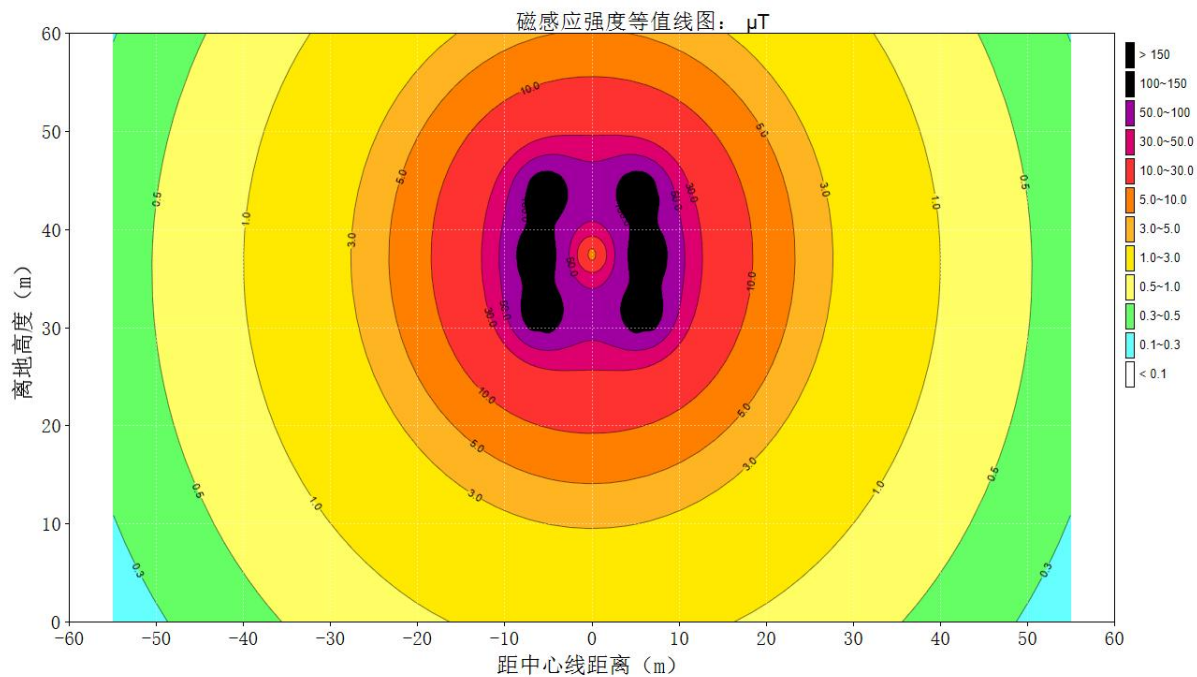
图 3-6 220kV 熟剑线新建段架空线路工频磁感应强度达标等值线图
