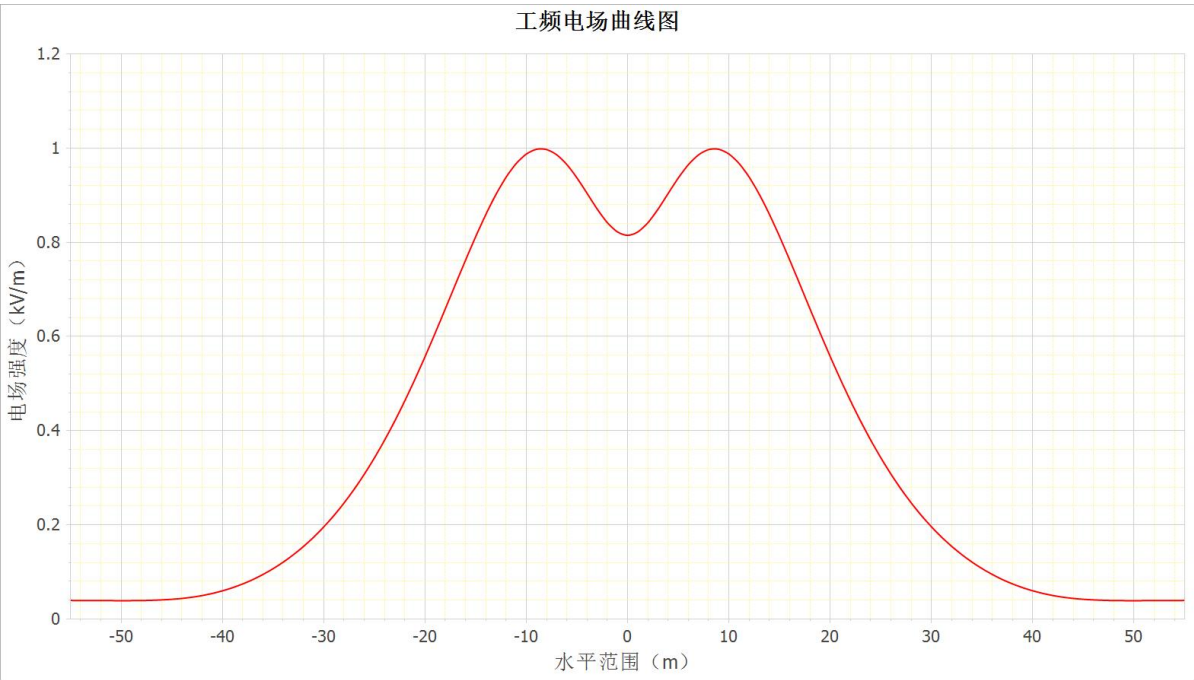
图 3-3 220kV 熟剑线恢复架线段架空线路下工频电场随距离变化趋势图
