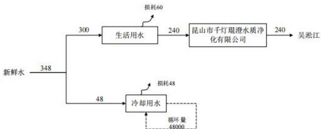
图 2-5 现有项目水平衡图 (单位: t/a)
