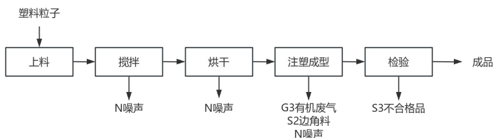
图 2-3 注塑成型生产工艺流程图
