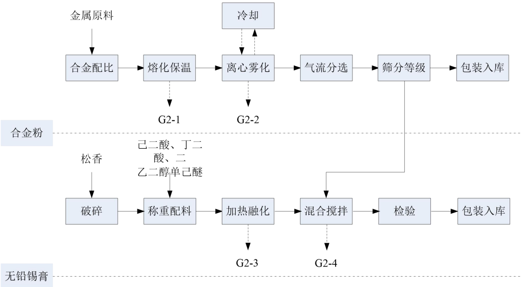
图 2-5 合金粉膏工艺流程及产污环节图
