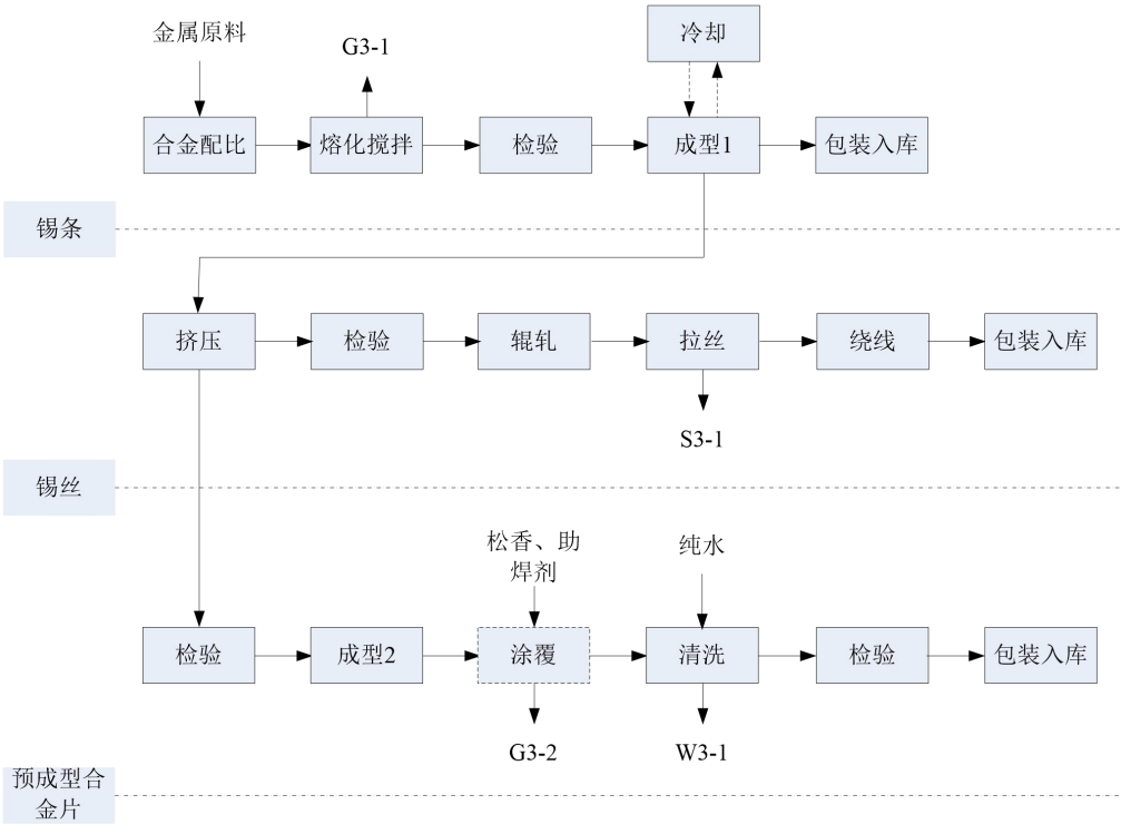
图 2-6 锡条、锡丝、预成型合金片生产工艺及产污环节流程图
