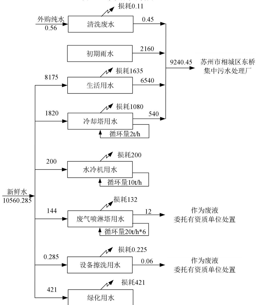
图 2-2 全厂水平衡图 (t/a)
