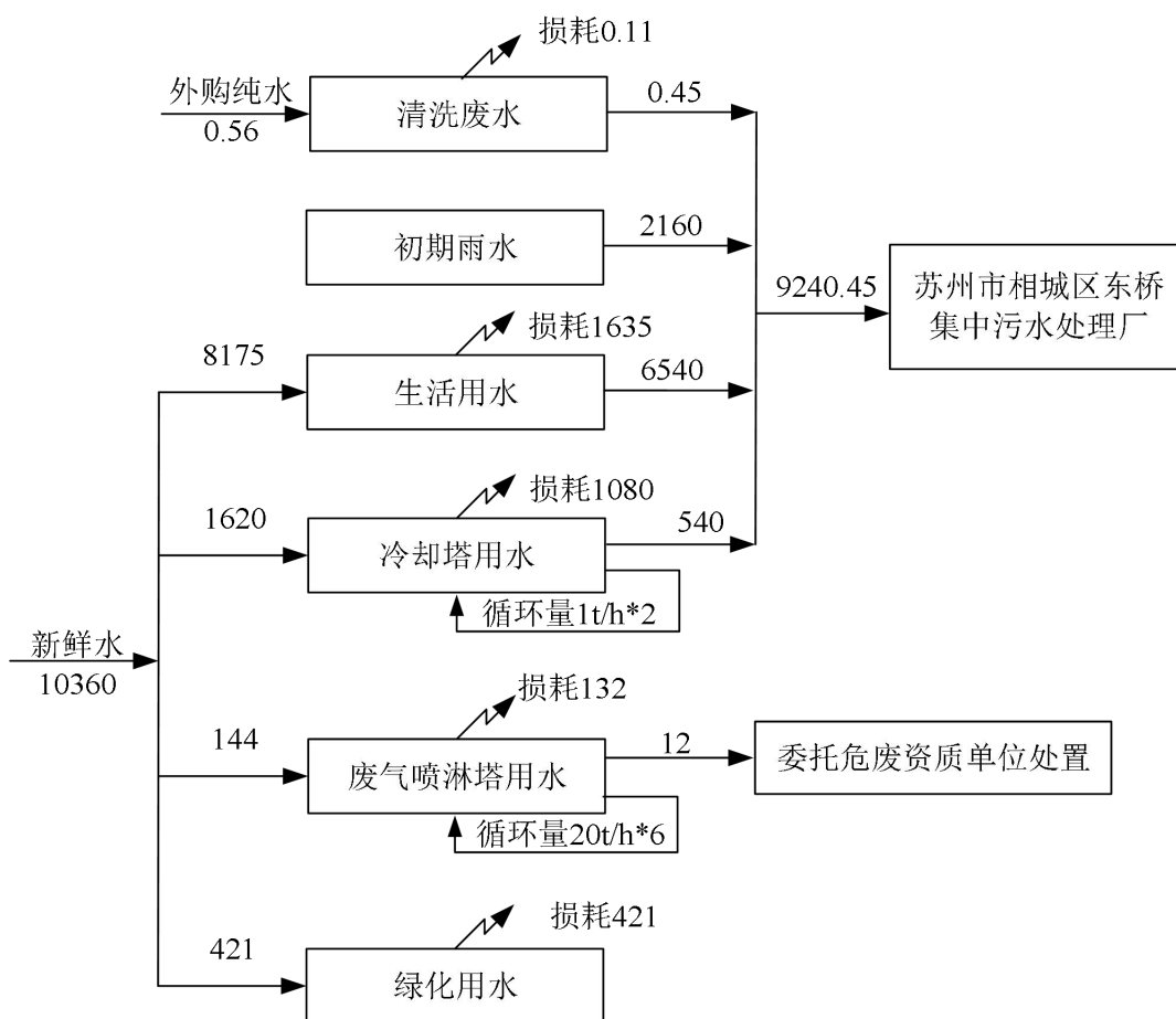
图 2-8 现有项目+在建项目水平衡图 (单位: \text{m}^3/\text{a} )
