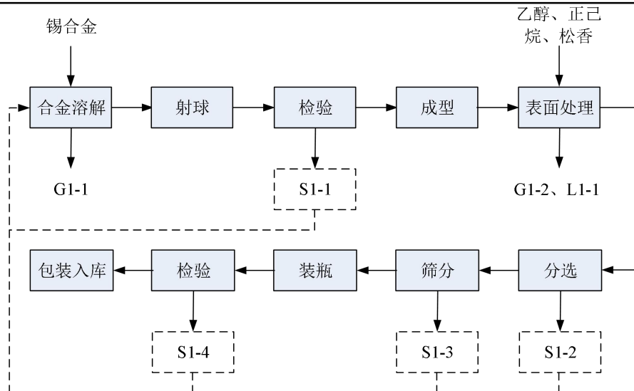
图 2-4 半导体用封装凸球工艺流程及产污节点
