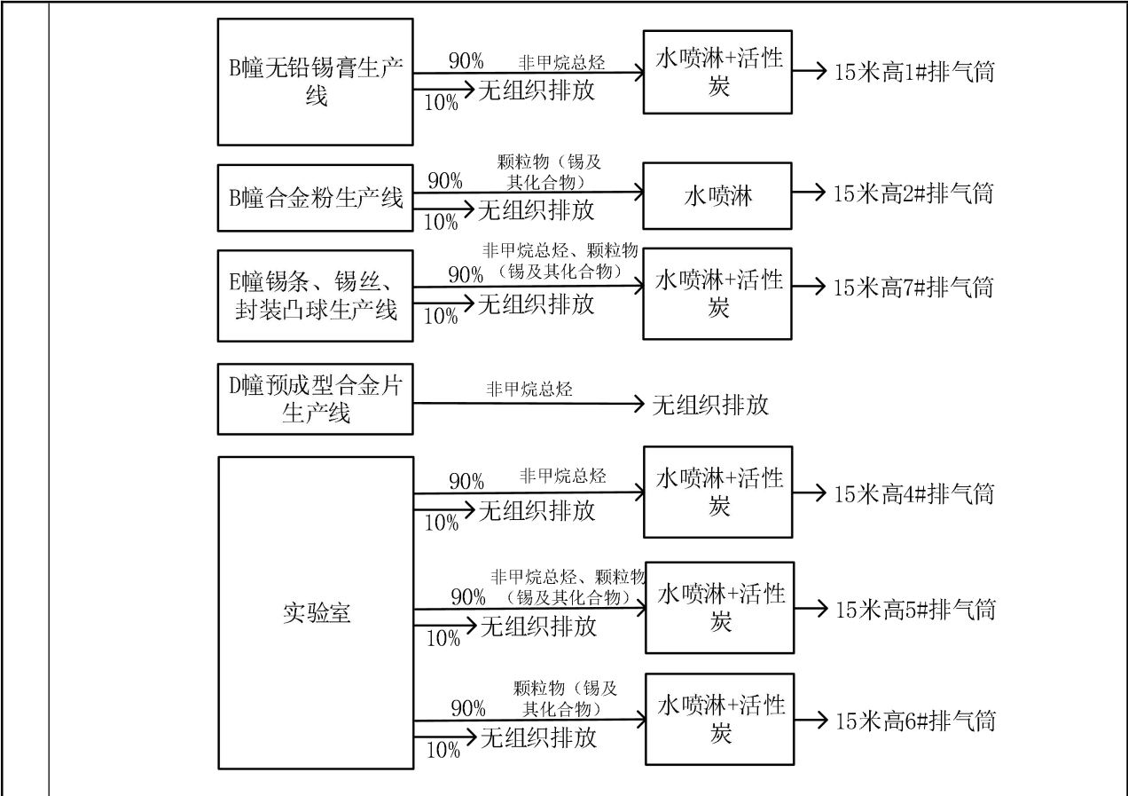
图 2-7 现有项目废气收集及处置情况
