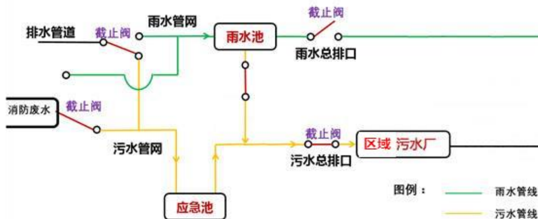
图 2-9 防止事故水进入外环境的控制、封堵系统图
