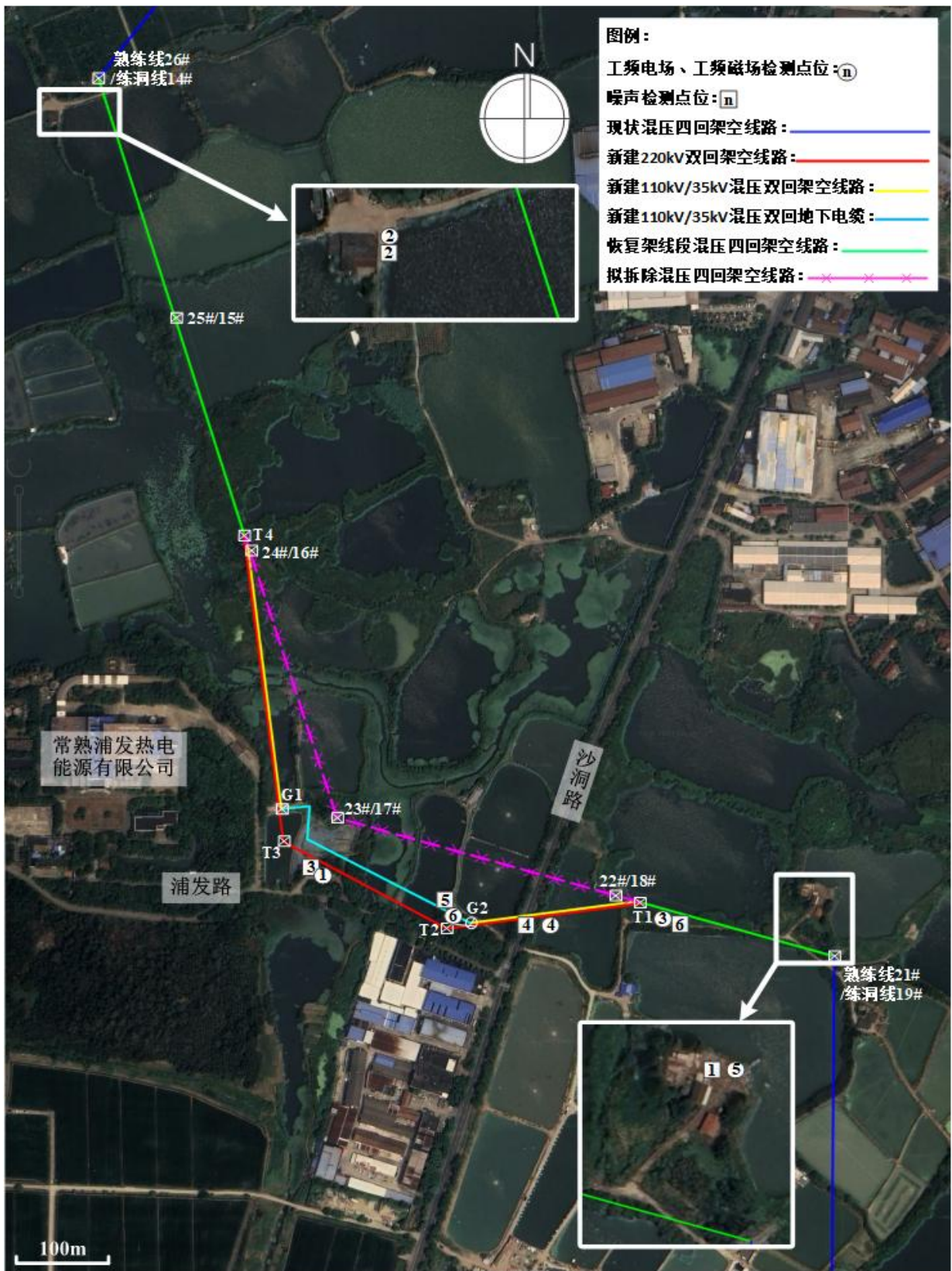
附图3 项目监测点位布置图
