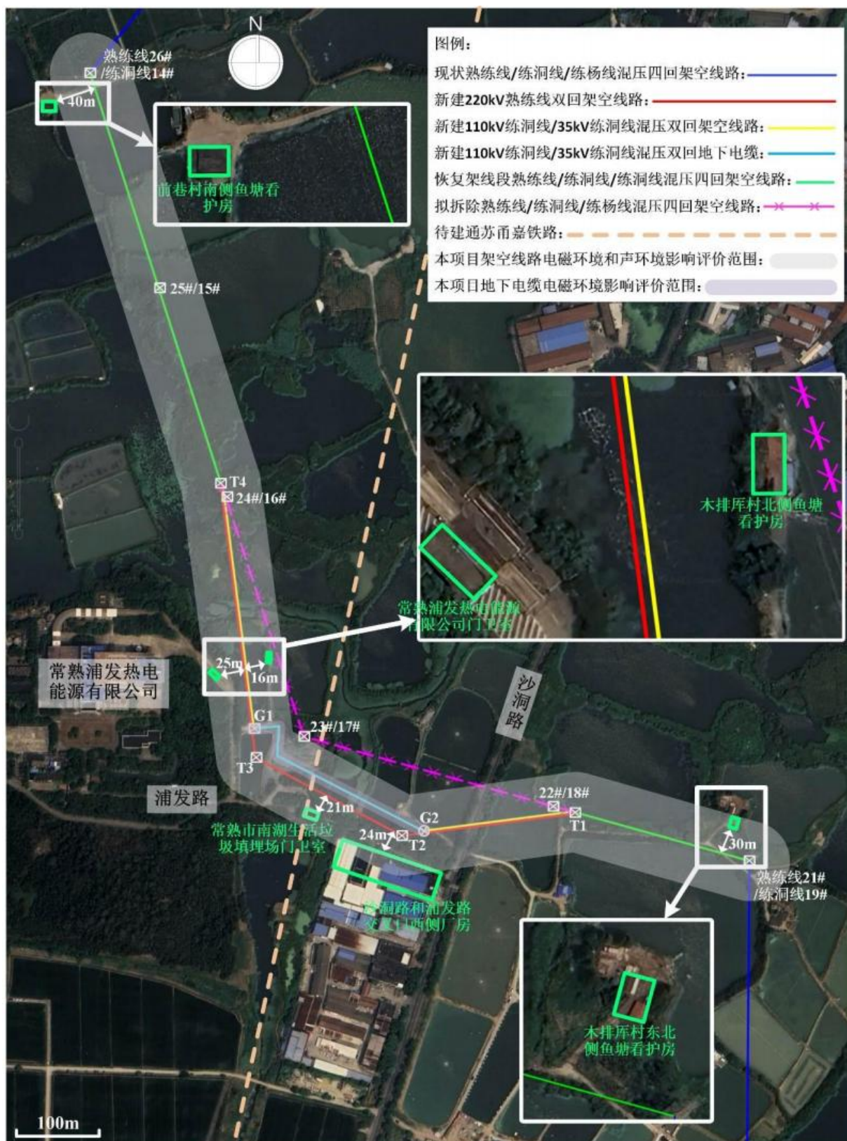
附图2 项目线路路径、周围环境及环境保护目标分布示意图
