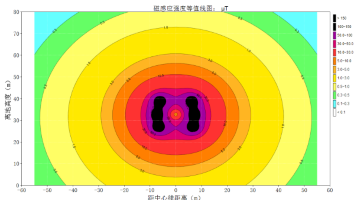
图 3-12 220kV 熟春 4X39/4X40 线双回架空线路工频磁感应强度达标等值线图
