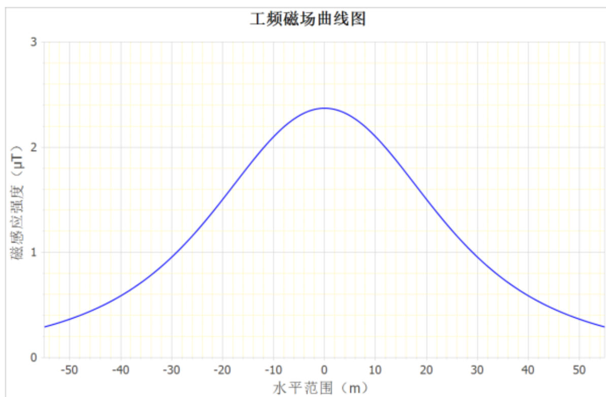
图 3-14 220kV 熟渭线/熟春线四回架空线路下工频磁场随距离变化趋势图
