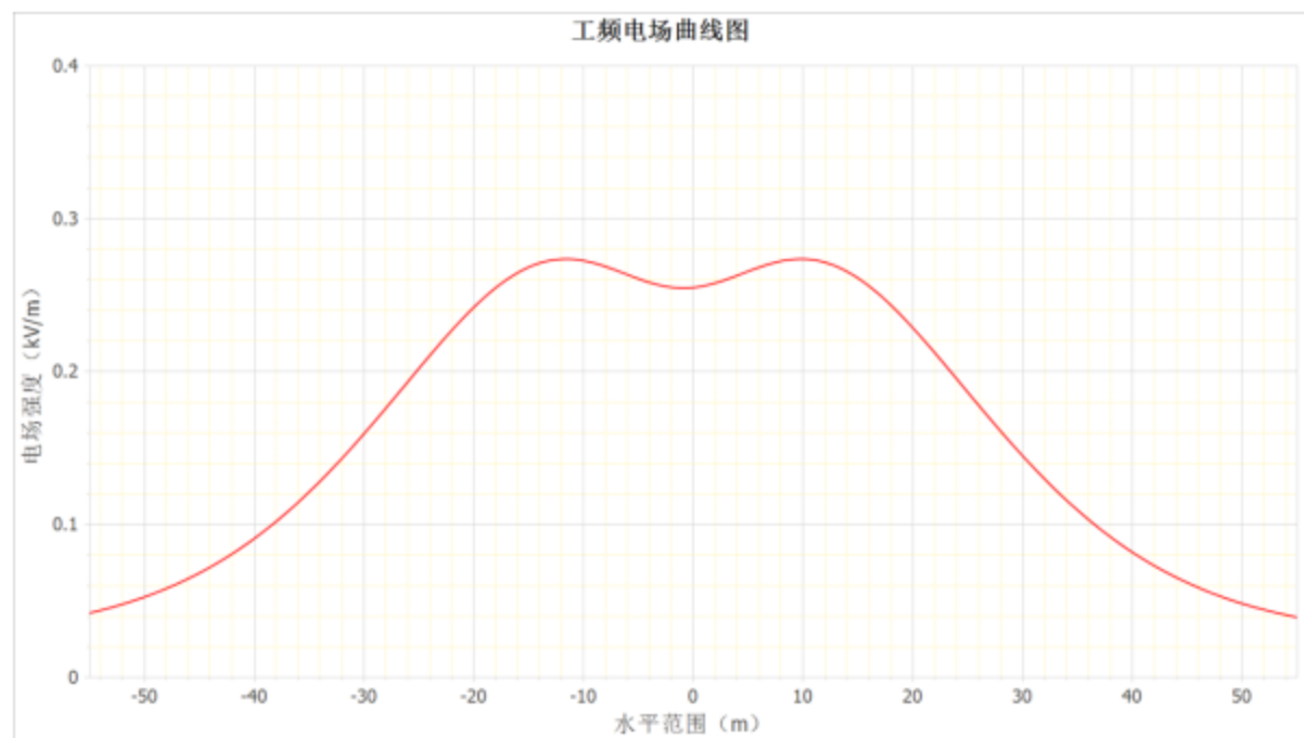
图 3-5 220kV 熟渭 4X37/4X38 线双回架空线路 (2S2-SJ4 塔型) 下工频电场随距离变化趋势图
