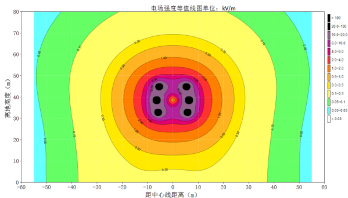
图 3-3 220kV 熟渭 4X37/4X38 线双回架空线路 (2S2-SJ1 塔型) 工频电场强度达标等值线图
