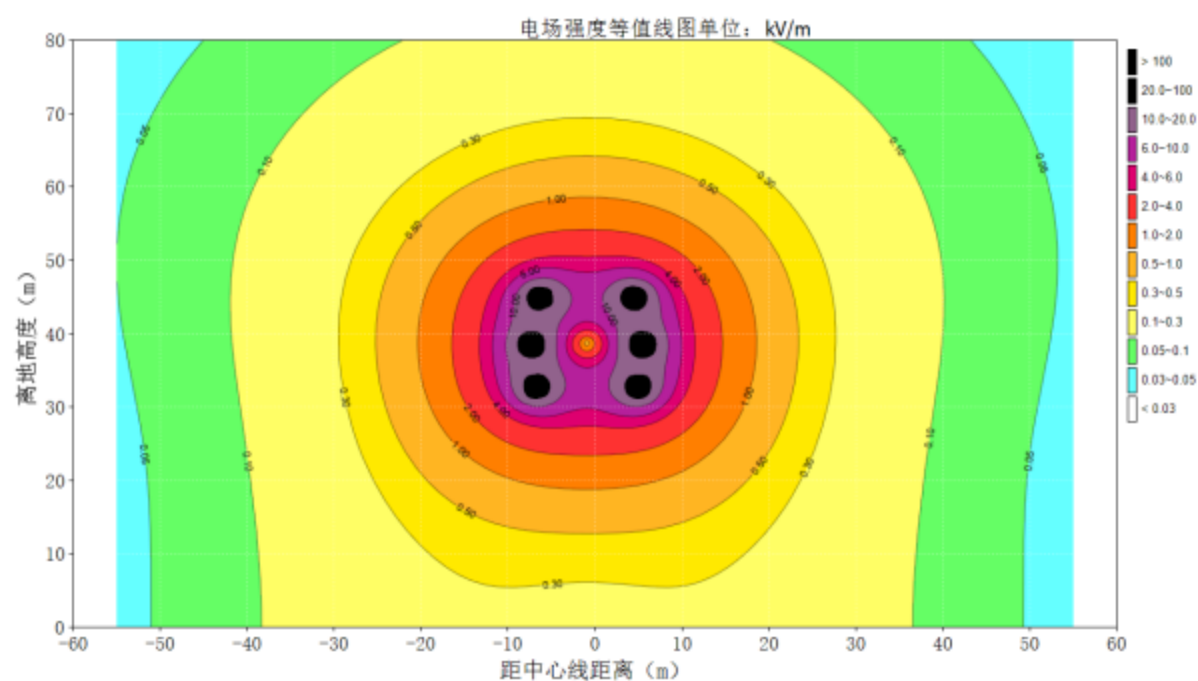
图 3-7 220kV 熟渭 4X37/4X38 线双回架空线路 (2S2-SJ4 塔型) 工频电场强度达标等值线图
