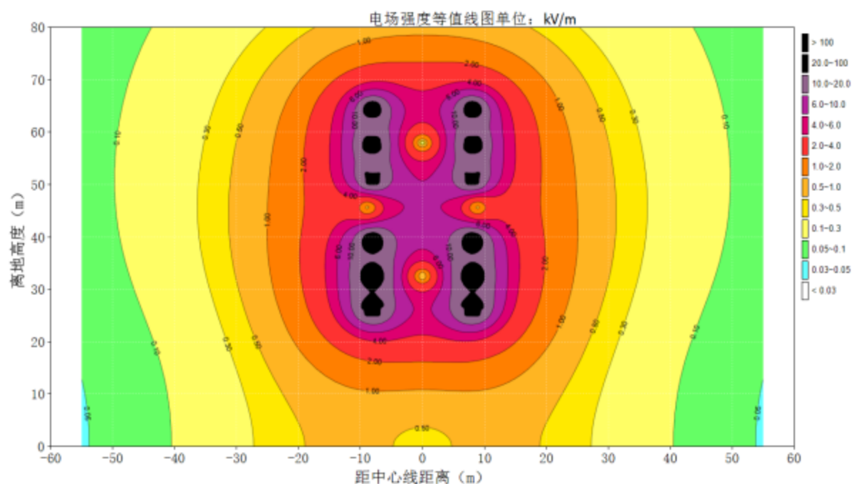
图 3-15 220kV 熟渭线/熟春线四回架空线路工频电场强度达标等值线图
