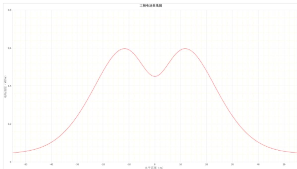
图 3-13 220kV 熟渭线/熟春线四回架空线路下工频电场随距离变化趋势图
