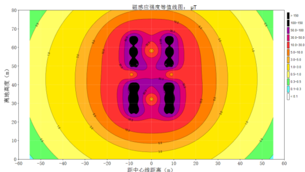
图 3-16 220kV 熟渭线/熟春线四回架空线路工频磁感应强度达标等值线图
