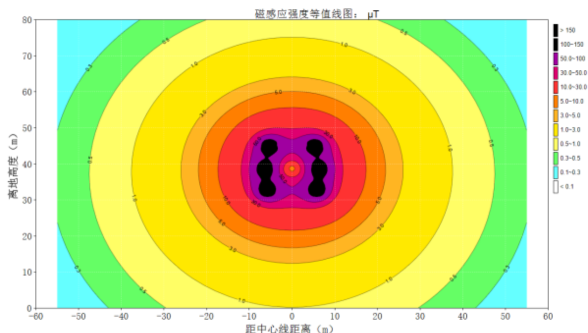
图 3-4 220kV 熟渭 4X37/4X38 线双回架空线路（2S2-SJ1 塔型）工频磁感应强度达标等值线图
