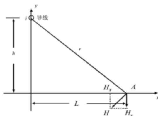
图 d 磁场向量图
