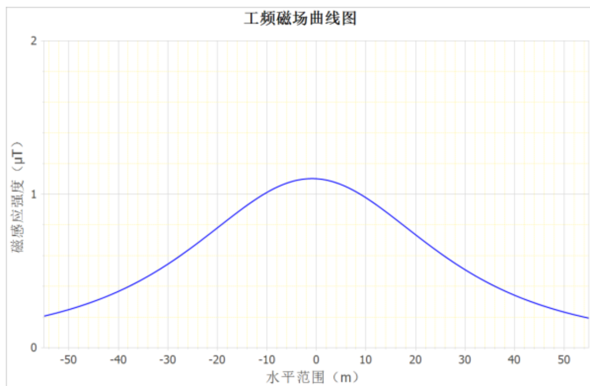
图 3-6 220kV 熟渭 4X37/4X38 线双回架空线路 (2S2-SJ4 塔型) 下工频磁场随距离变化趋势图
