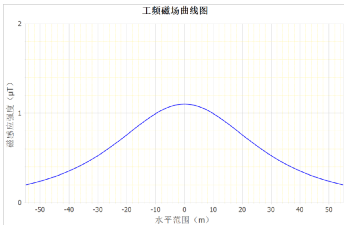
图 3-2 220kV 熟渭 4X37/4X38 线双回架空线路 (2S2-SJ1 塔型) 下工频磁场随距离变化趋势图
