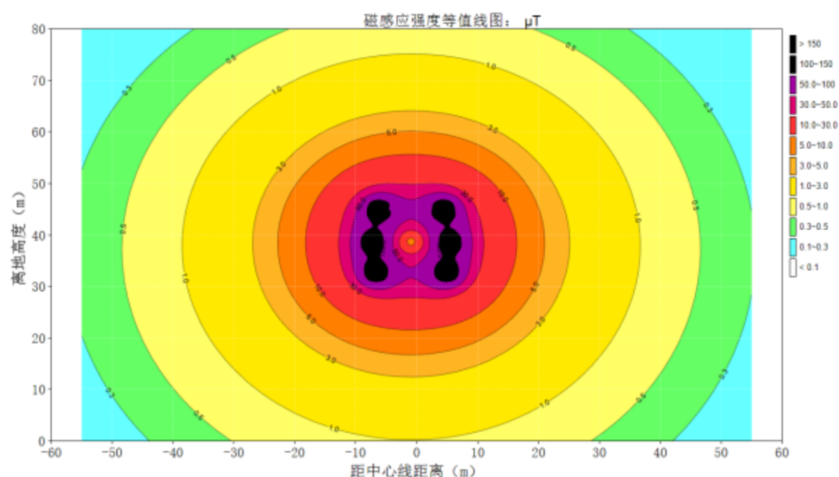
图 3-8 220kV 熟渭 4X37/4X38 线双回架空线路（2S2-SJ4 塔型）工频磁感应强度达标等值线图
