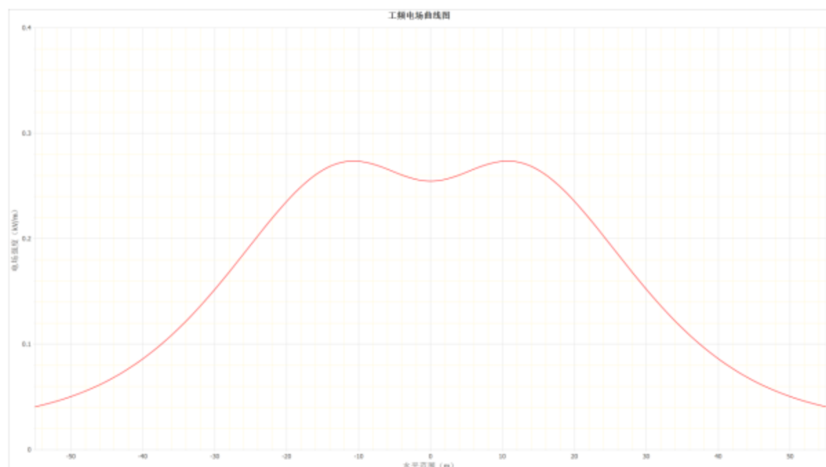
图 3-1 220kV 熟渭 4X37/4X38 线双回架空线路 (2S2-SJ1 塔型) 下工频电场随距离变化趋势图
