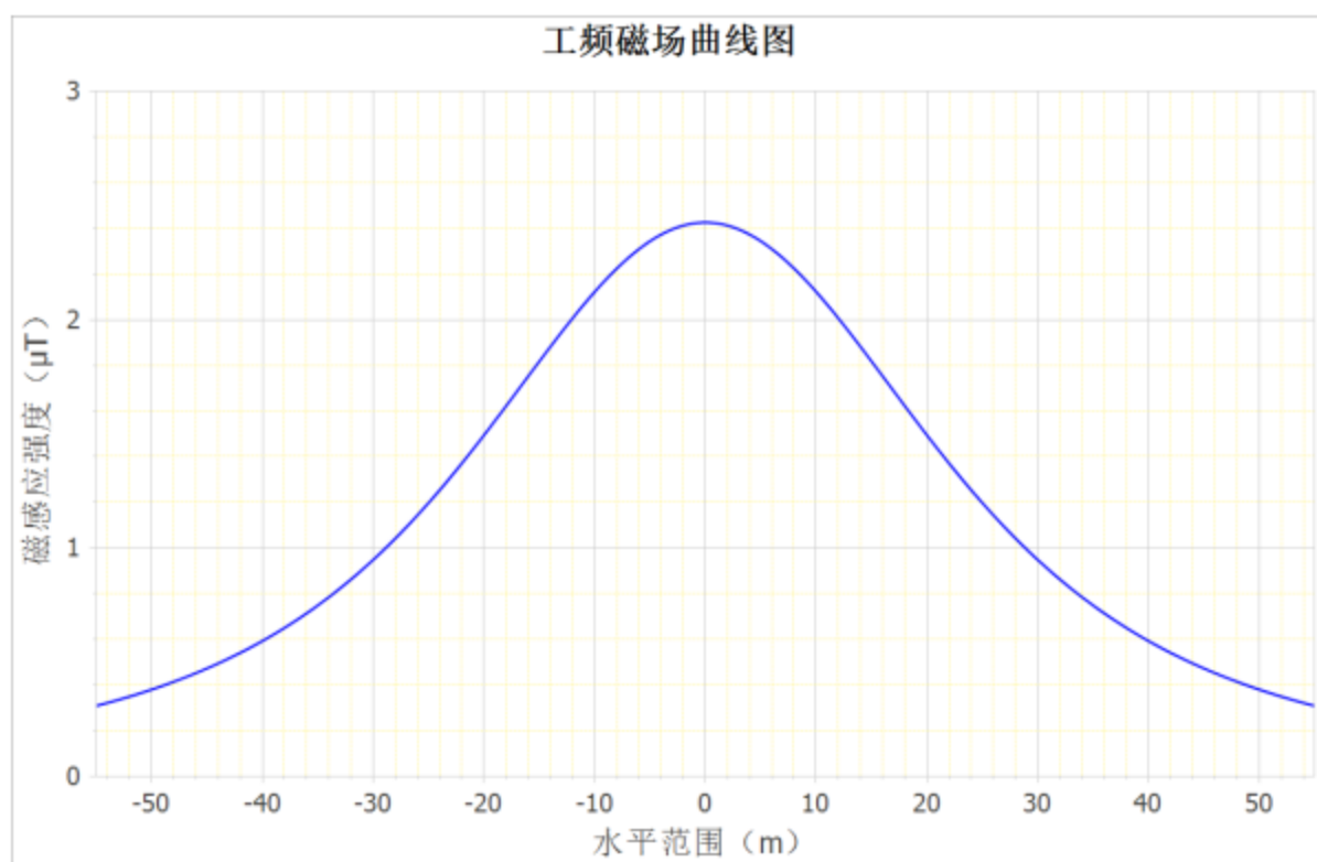
图 3-10 220kV 熟春 4X39/4X40 线双回架空线路下工频磁场随距离变化趋势图
