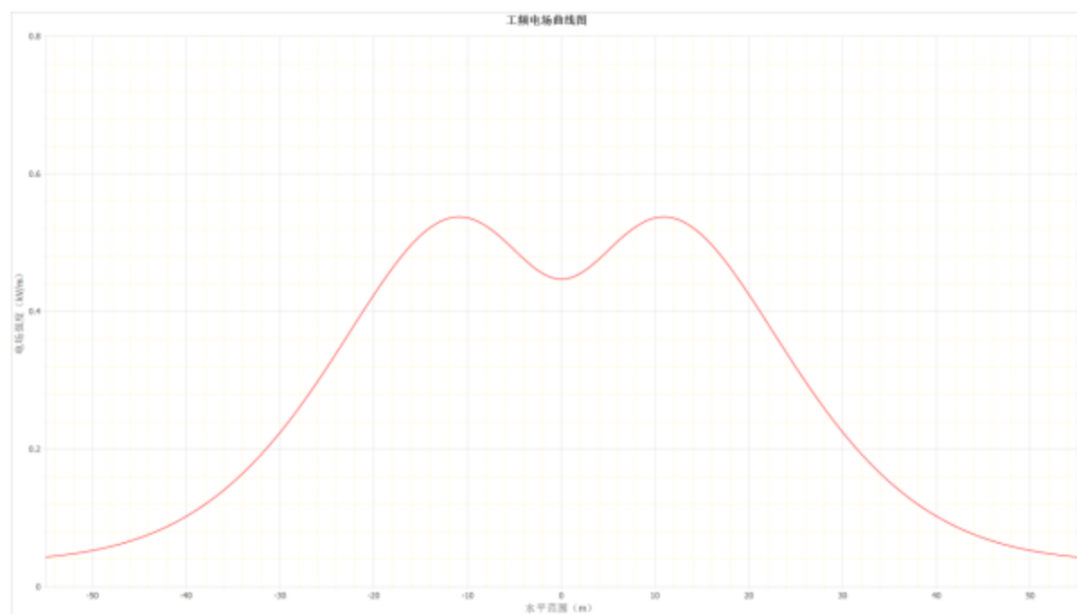
图 3-9 220kV 熟春 4X39/4X40 线双回架空线路下工频电场随距离变化趋势图
