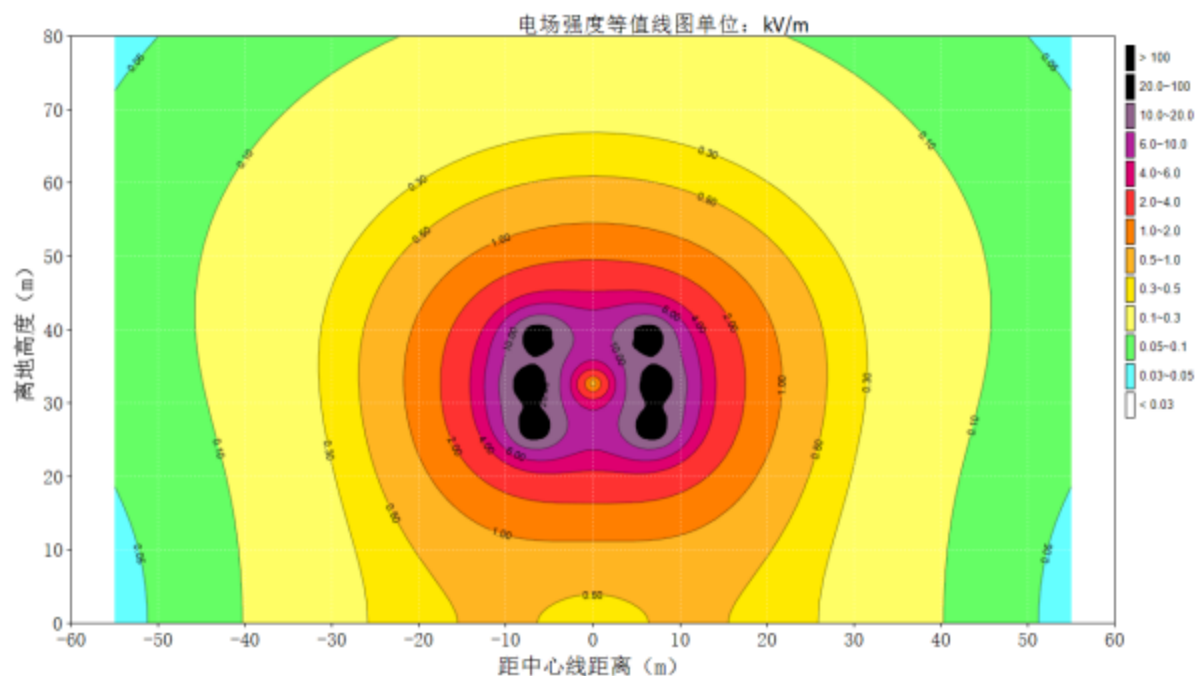
图 3-11 220kV 熟春 4X39/4X40 线双回架空线路工频电场强度达标等值线图
