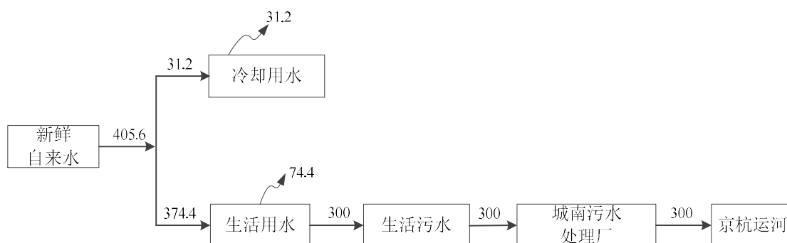
图 2-2 本项目水平衡图
