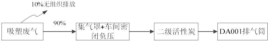
图4-1 废气收集、处理、排放流程图
