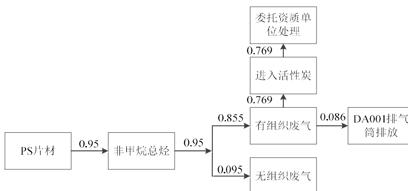
图 2-1 本项目 VOCs 平衡图
