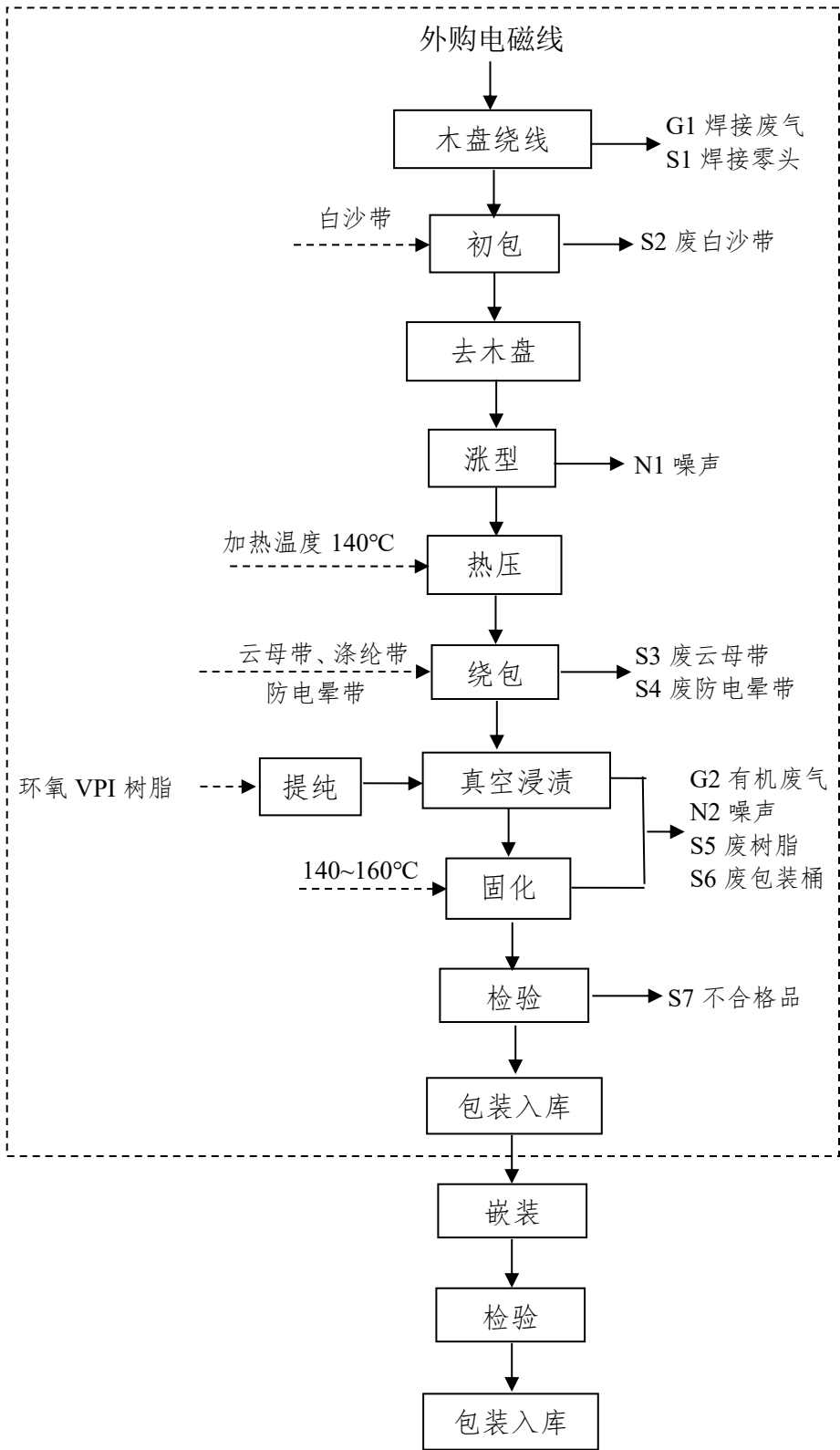
图 2-1 高压电机线圈、高压绝缘系统生产工艺流程
