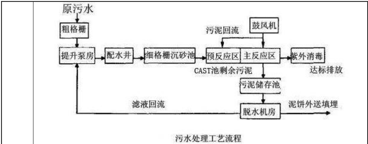
图 4-6 芦墟污水处理厂废水处理工艺流程图
