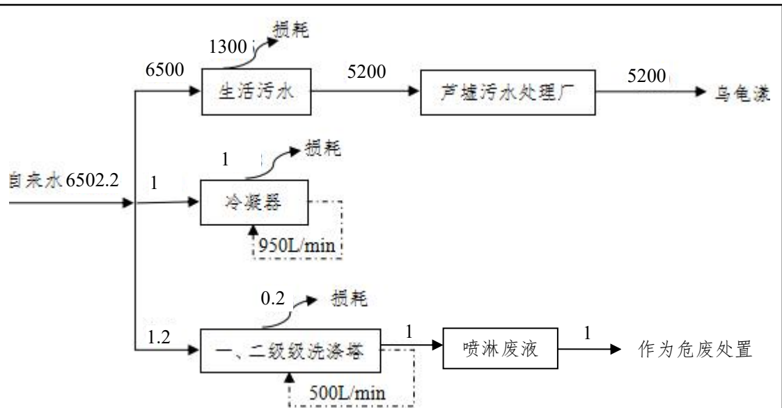
图 4-4 本项目水平衡图 (t/a)
