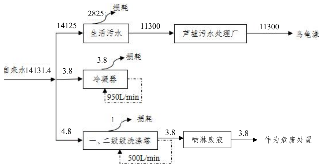
图 4-5 扩建后全厂水平衡图 (t/a)
