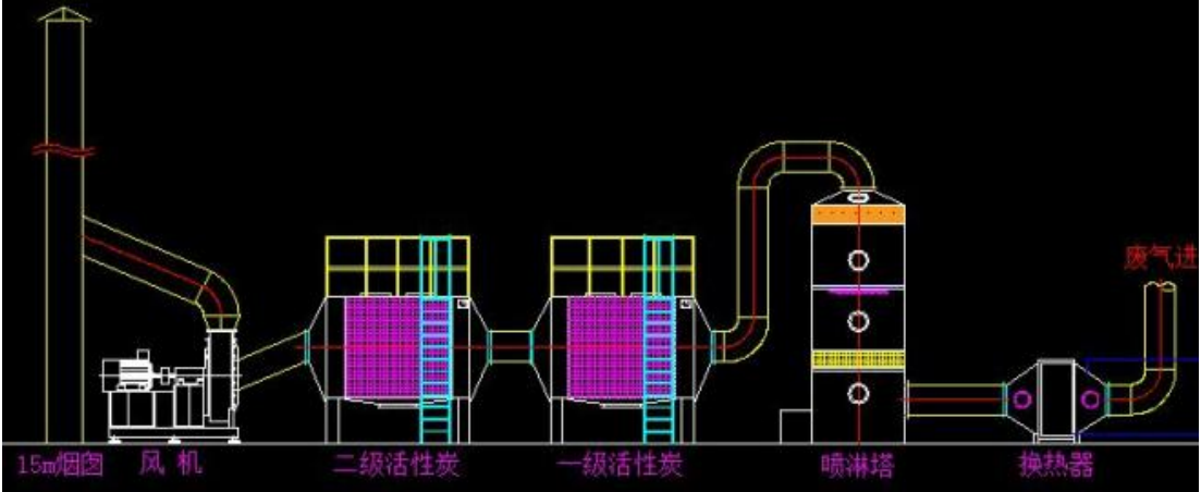
图 4-2 换热器+水洗塔+除雾箱+活性炭吸附装置工艺流程图
