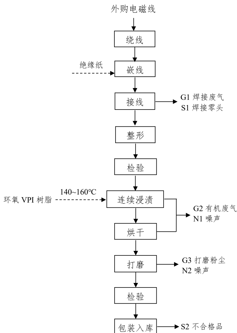
图 2-3 电机线圈（低压）生产工艺流程图
