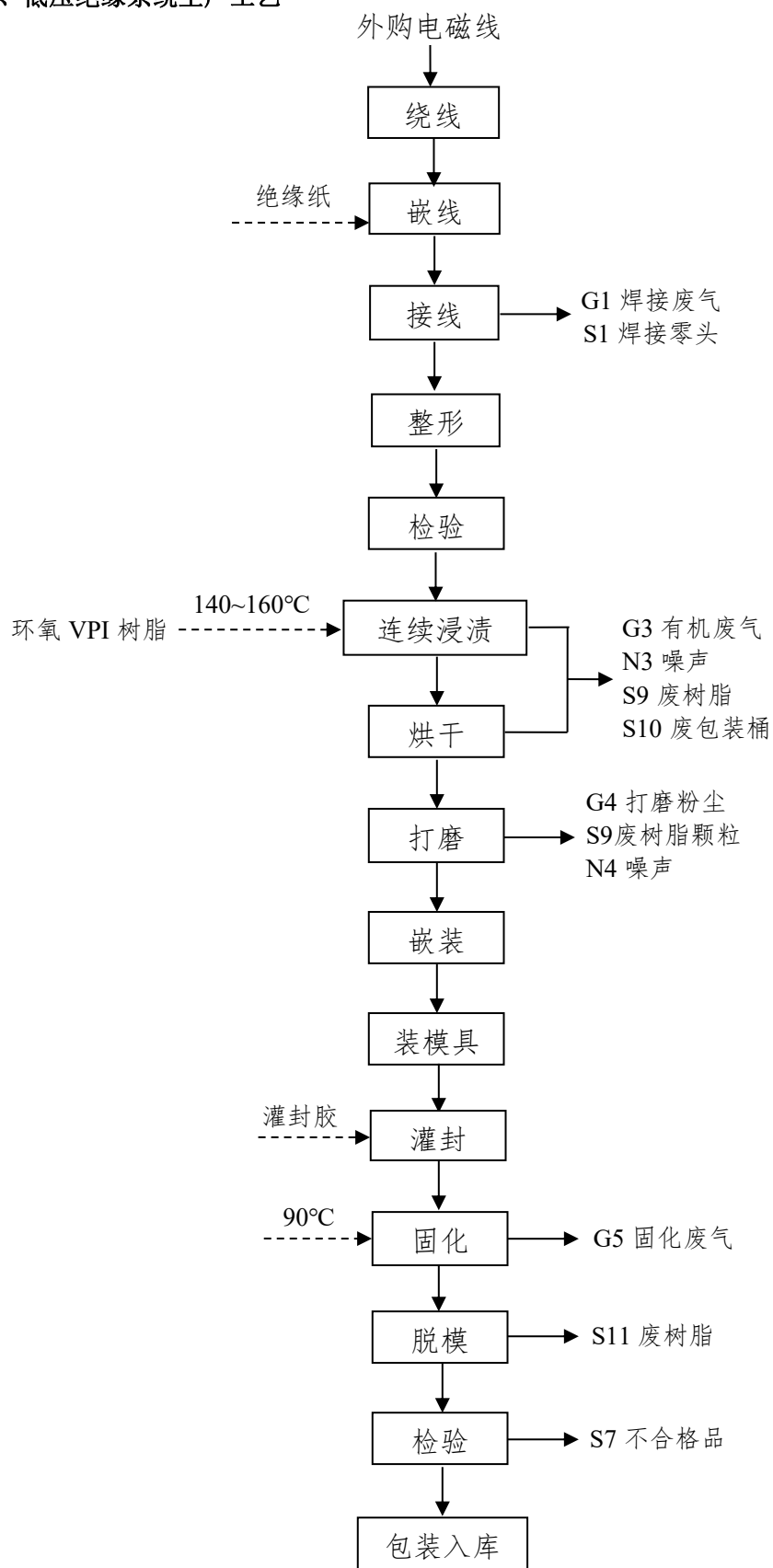
图 2-2 低压绝缘系统生产工艺流程
