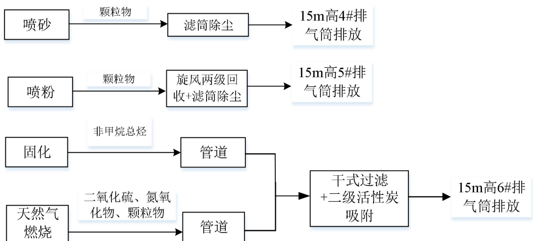
图 4-1 本项目废气收集处理流程图
