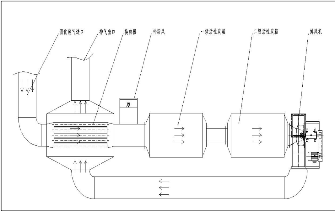
图 4-3 固化废气处理设施原理图
