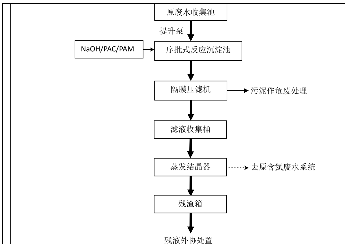
图 4-8 蒸发结晶工艺流程图
