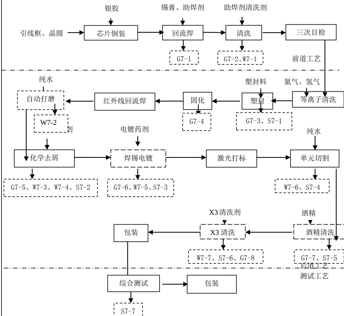
图 2-12 倒装 MLP 工艺流程图
