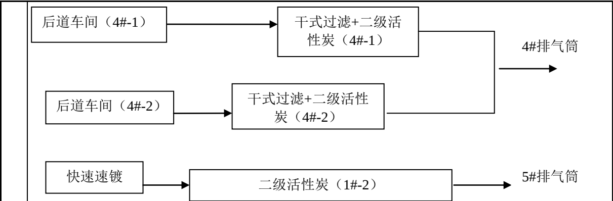
图 2-19 现有项目废气收集处理汇总
