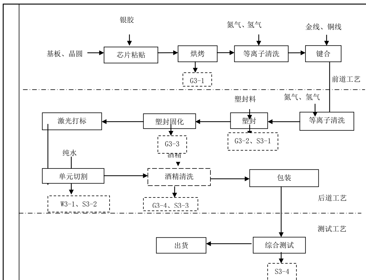
图 2-8 传统正装 LGA 工艺流程图
