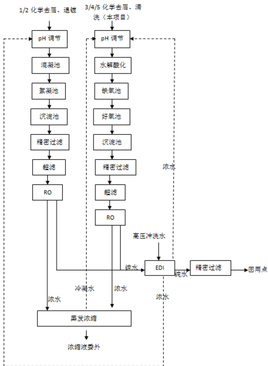
图 4-7 氮磷废水处理设施流程图
