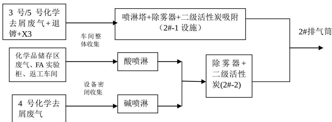
图 4-1 现有项目 2#排气筒处理设施情况
