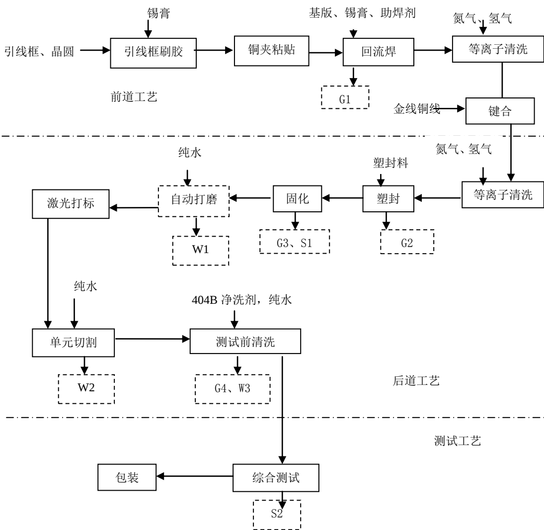
图 2-3 铜夹类 MLP 工艺流程图
