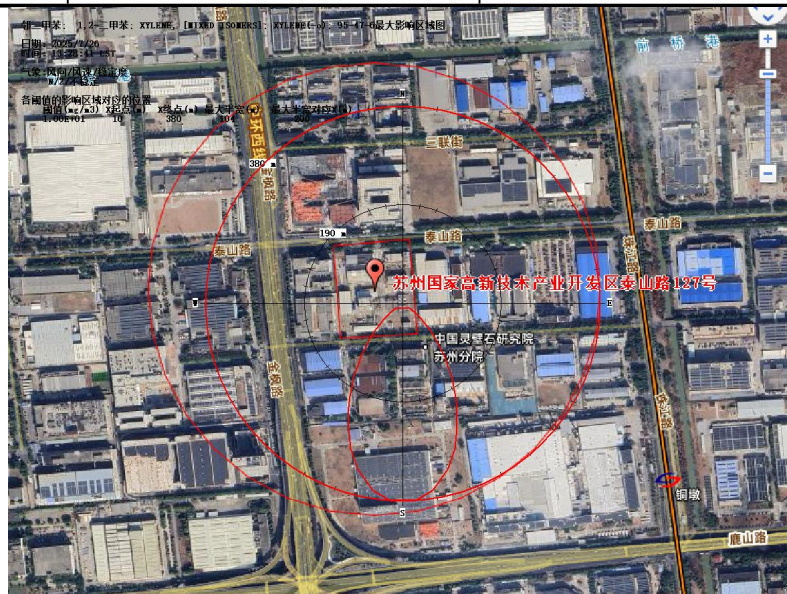
图 6.2-2 二甲苯储罐泄漏事故各阈值的廓线
