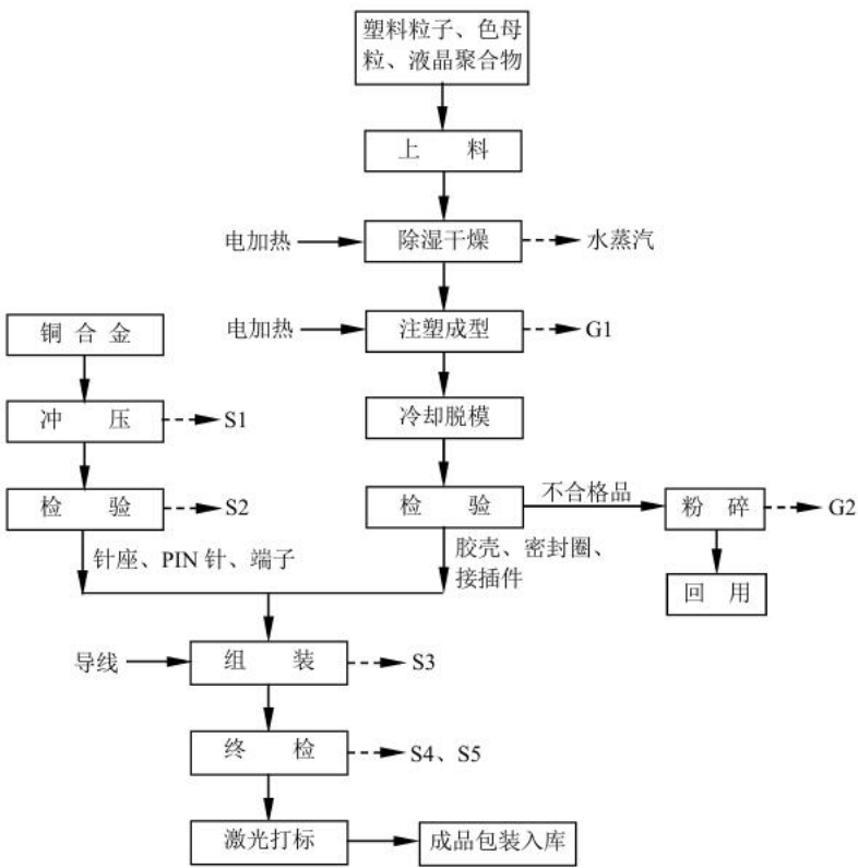
图 2-7 现有项目连接器、特种线束生产工艺流程图
