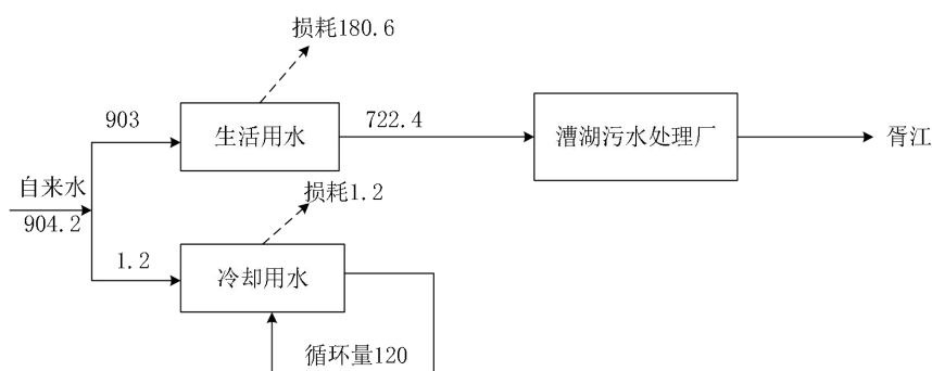
图 2-3 本项目水平衡图（单位：t/a）
