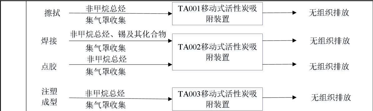
图 4-1 废气收集处理流程图
