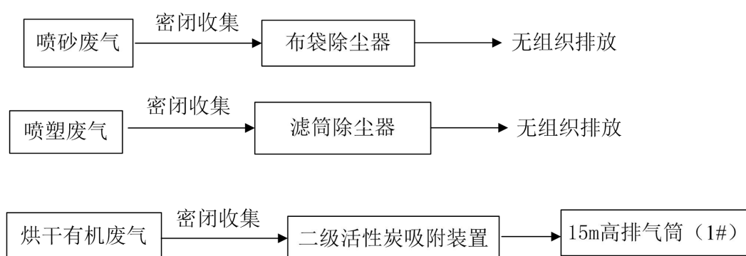
图 4-1 废气收集管线示意图
