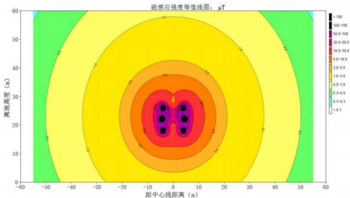
图 3-4 110kV 谢师 1788 线赵市支线新建段架空线路工频磁感应强度达标等值线图
