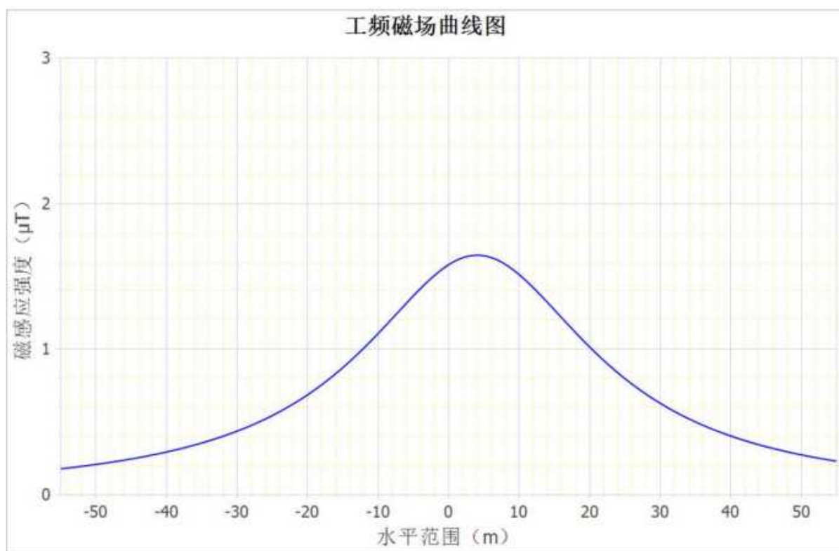
图3-6 110kV 谢师1788线赵市支线恢复架线段架空线路下工频磁场随距离变化趋势图
