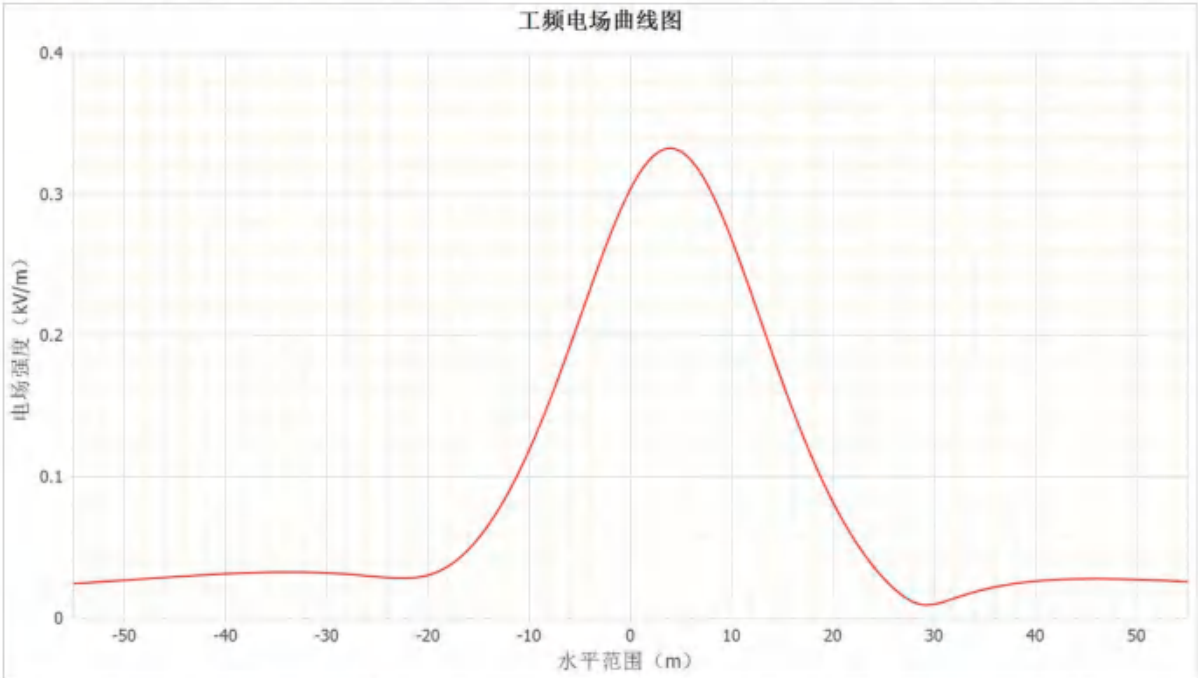
图 3-5 110kV 谢师 1788 线赵市支线恢复架线段架空线路下工频电场随距离变化趋势图
