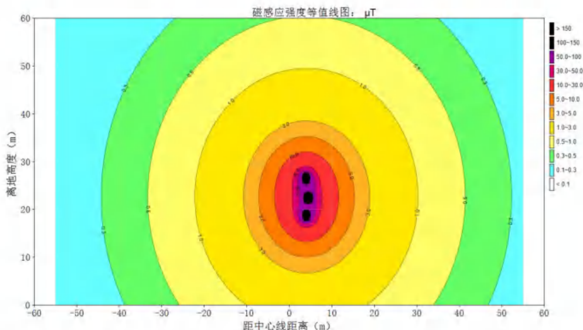
图3-8 110kV 谢师1788 线赵市支线恢复架线段架空线路工频磁感应强度达标等值线图
