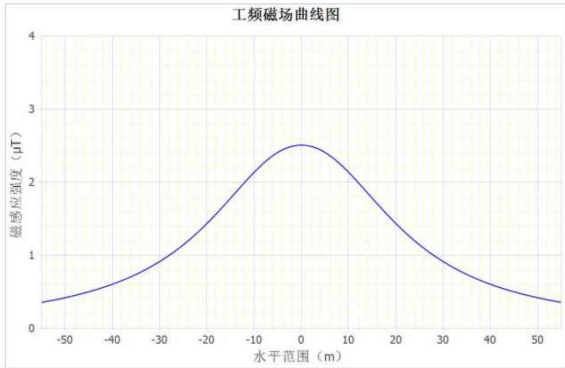
图 3-2 110kV 谢师 1788 线赵市支线新建段架空线路下工频磁场随距离变化趋势图
