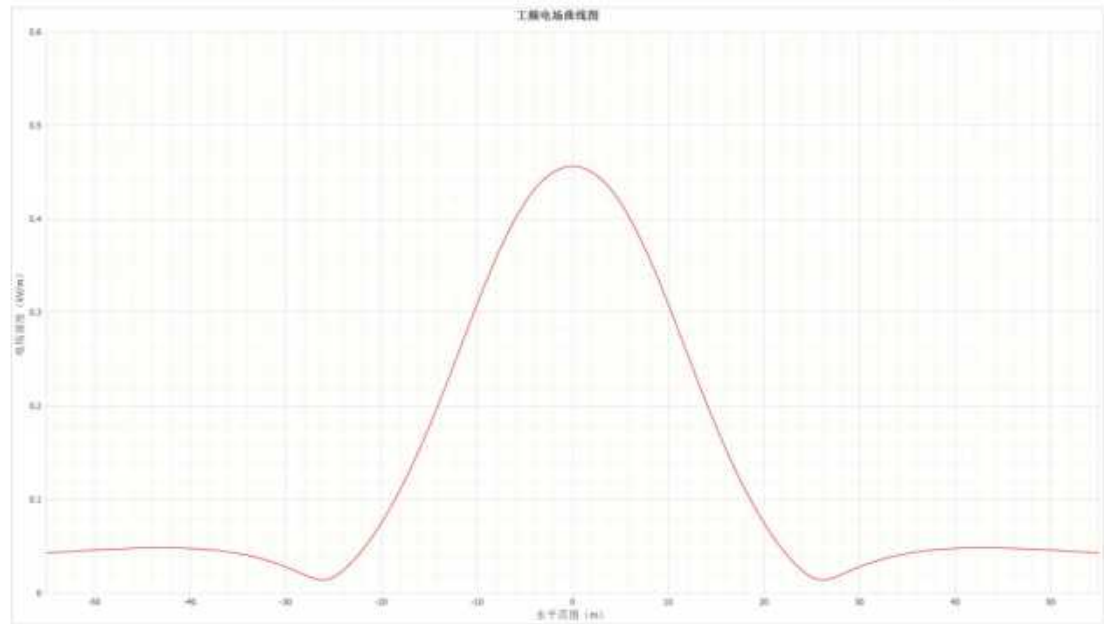
图 3-1 110kV 谢师 1788 线赵市支线新建段架空线路下工频电场随距离变化趋势图
