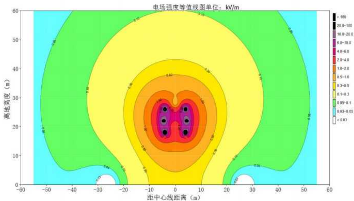
图 3-3 110kV 谢师 1788 线赵市支线新建段架空线路工频电场强度达标等值线图
