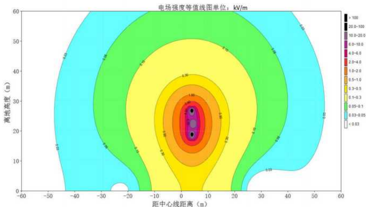
图3-7 110kV 谢师1788线赵市支线恢复架线段架空线路工频电场强度达标等值线图
