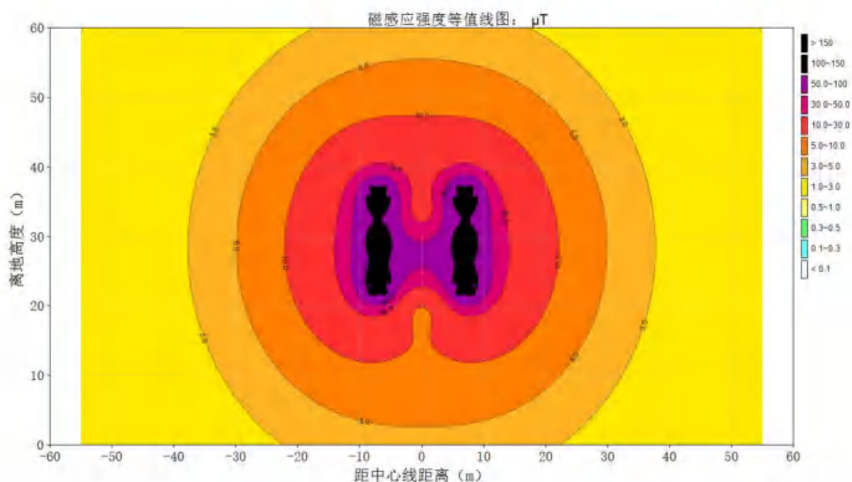
图 3-8 220kV 常谢/常同线恢复架线段架空线路工频磁感应强度达标等值线图
