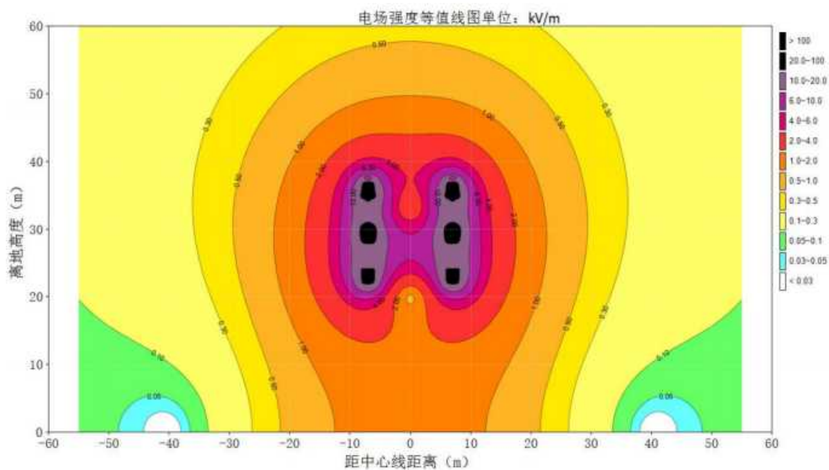
图 3-7 220kV 常谢/常同线恢复架线段架空线路工频电场强度达标等值线图
