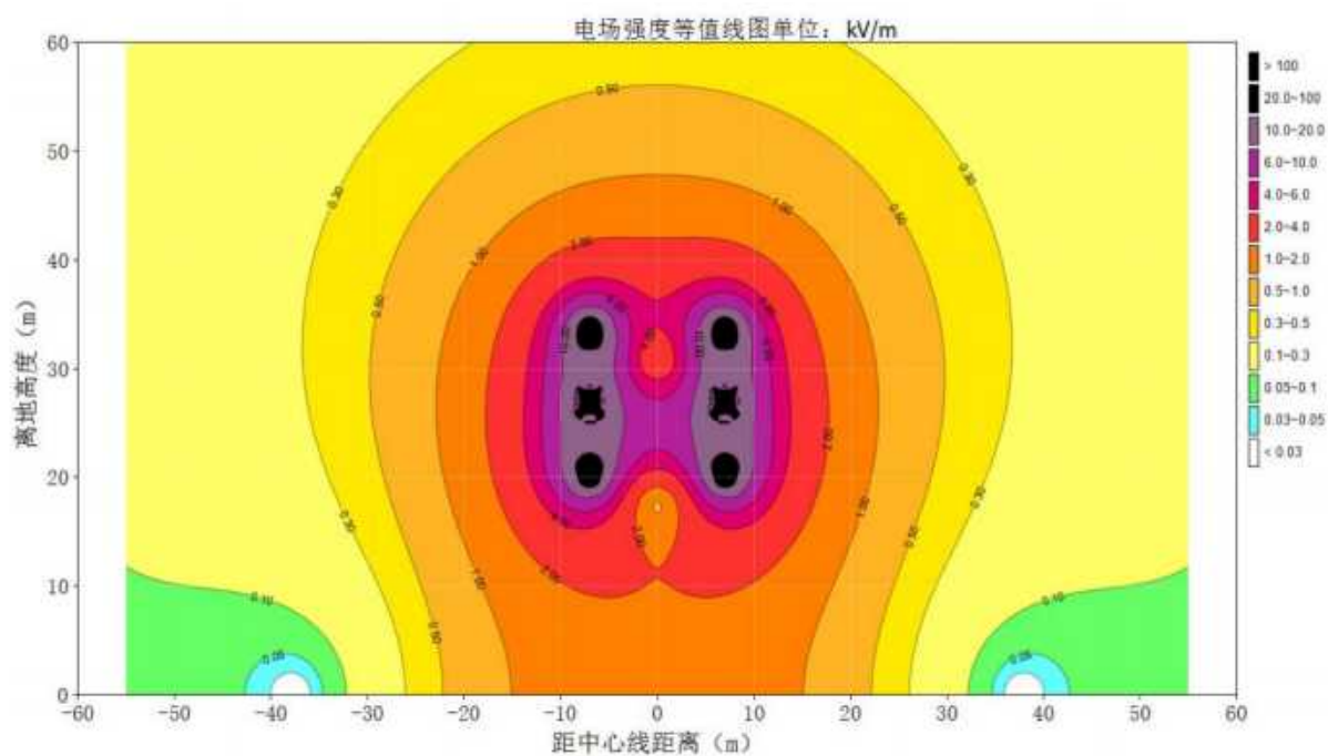
图 3-3 220kV 常谢/常同线新建段架空线路工频电场强度达标等值线图
