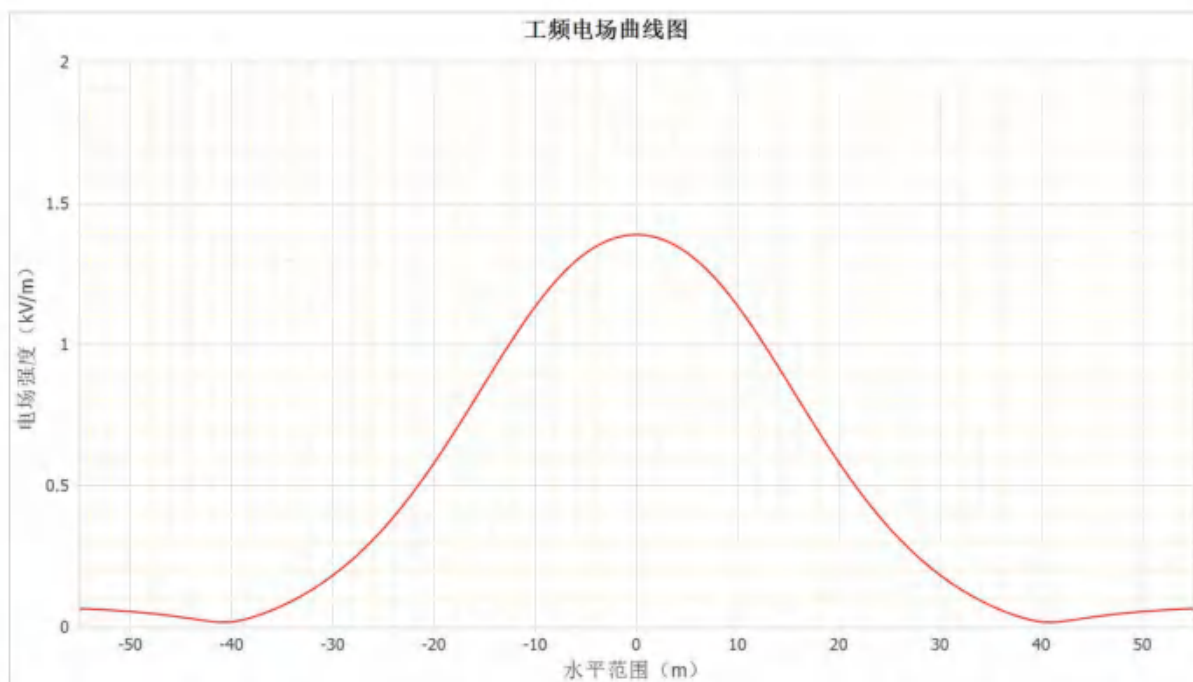
图 3-5 220kV 常谢/常同线恢复架线段架空线路下工频电场随距离变化趋势图
