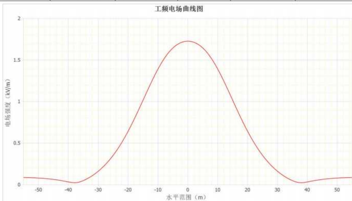
图 3-1 220kV 常谢/常同线新建段架空线路下工频电场随距离变化趋势图
