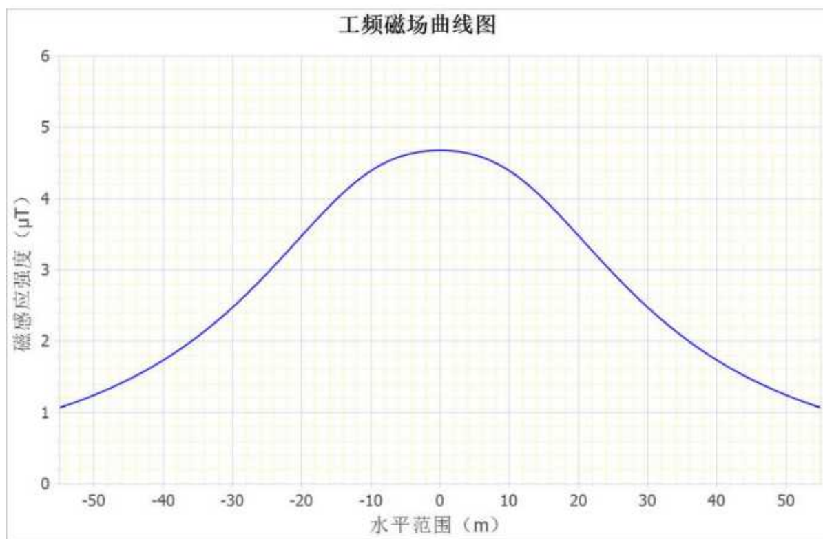
图 3-6 220kV 常谢/常同线恢复架线段架空线路下工频磁场随距离变化趋势图
