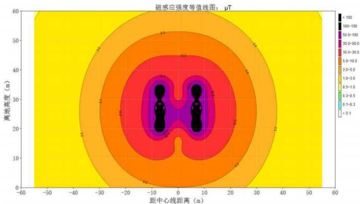
图 3-4 220kV 常谢/常同线新建段架空线路工频磁感应强度达标等值线图
