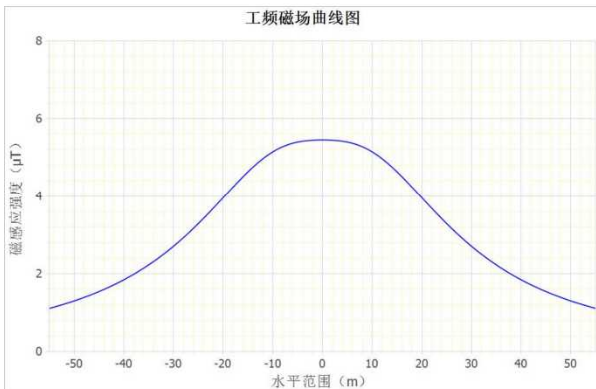
图 3-2 220kV 常谢/常同线新建段架空线路下工频磁场随距离变化趋势图
