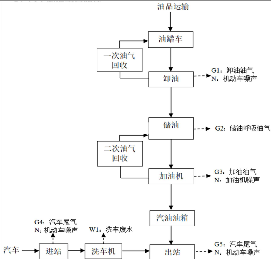
图 2-3 加油站工艺流程及产污环节图 (G-废气; W-废水; N-噪声)
