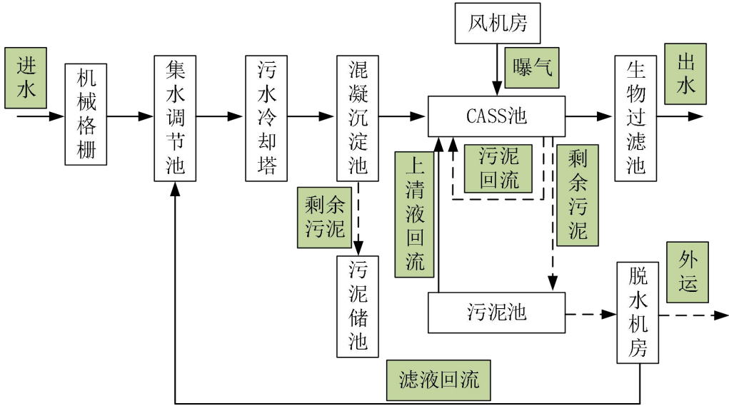
图 4-2 苏州高新区白荡水质净化厂工艺流程图
