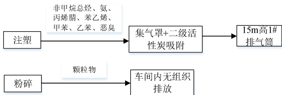
图 4-1 本项目废气收集处理流程图
