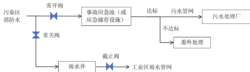
图 4-3 事故废水控制、封堵系统示意图
