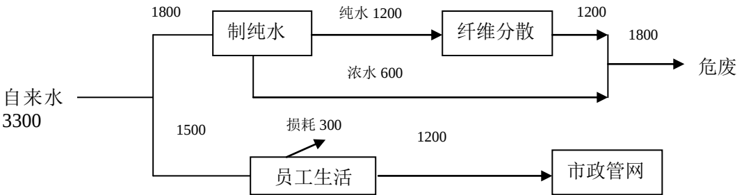
图 2-1 项目水平衡（t/a）
