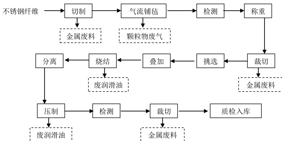
图 2-3 不锈钢纤维毡生产工艺流程图
