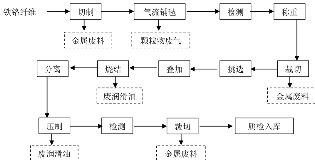
图 2-4 柴油过滤毡生产工艺流程图
