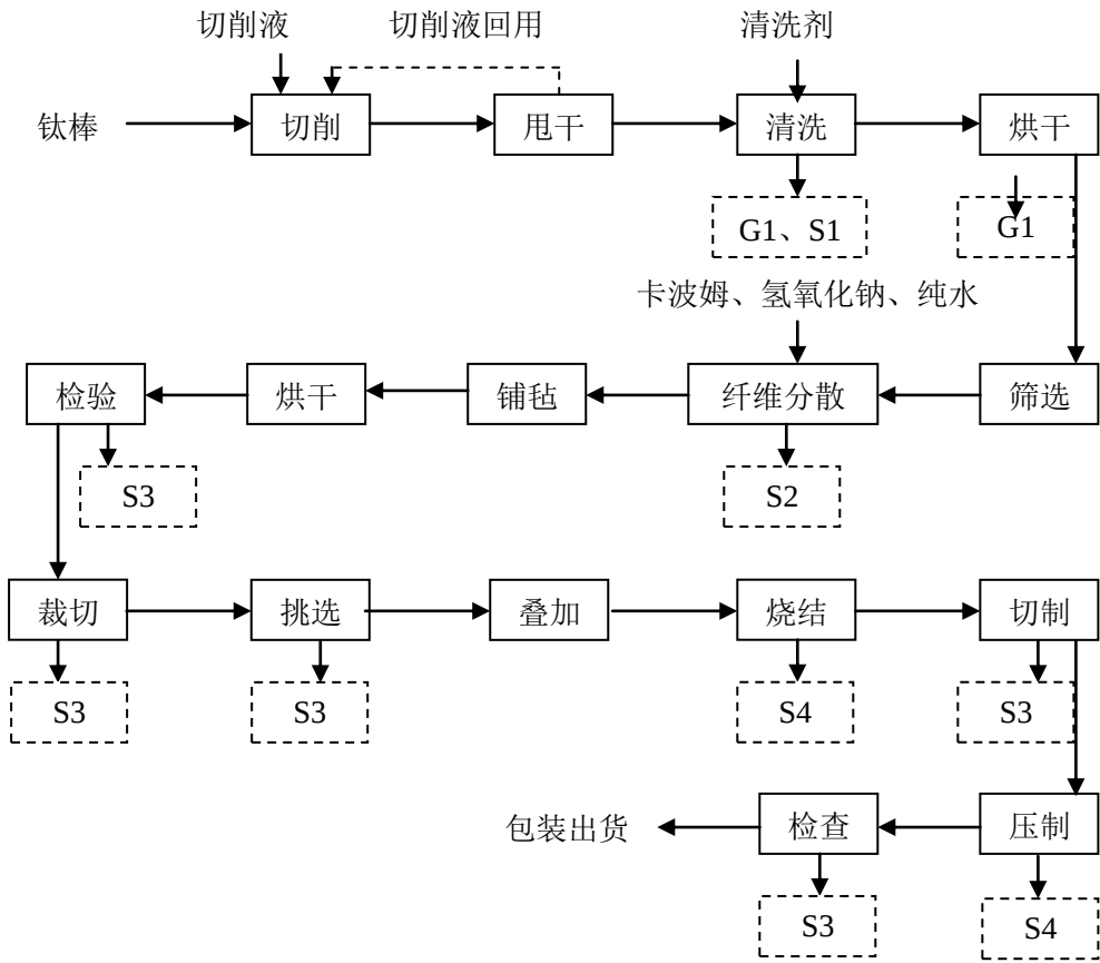
图 2-1 钛纤维烧结毡生产工艺流程图
