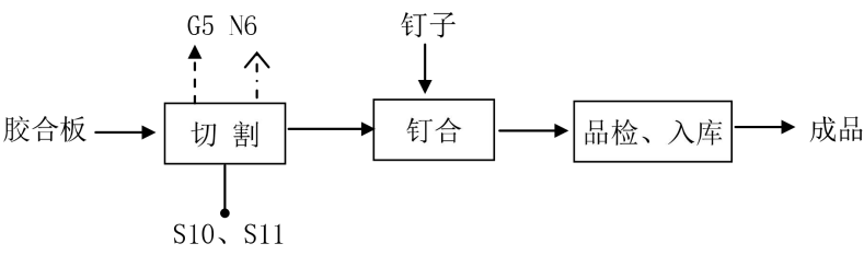
图 2-4 木制品生产工艺流程图
