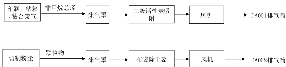
图 4-1 废气收集处理工艺流程图
