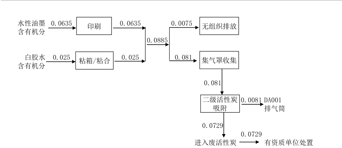
图 2-1 本项目非甲烷总烃物料平衡图 (t/a)
