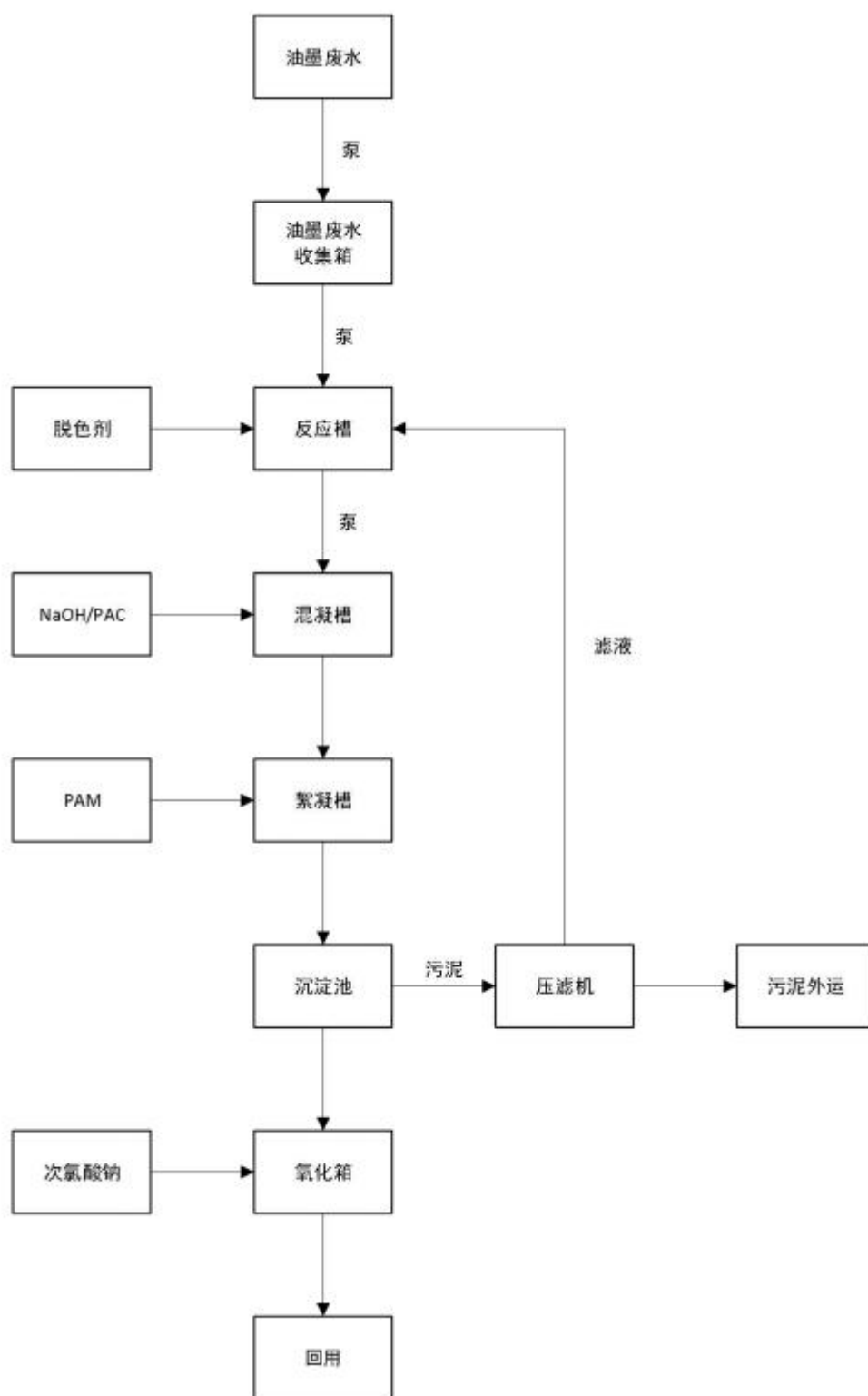
图 4-2 废水处理工艺流程图
