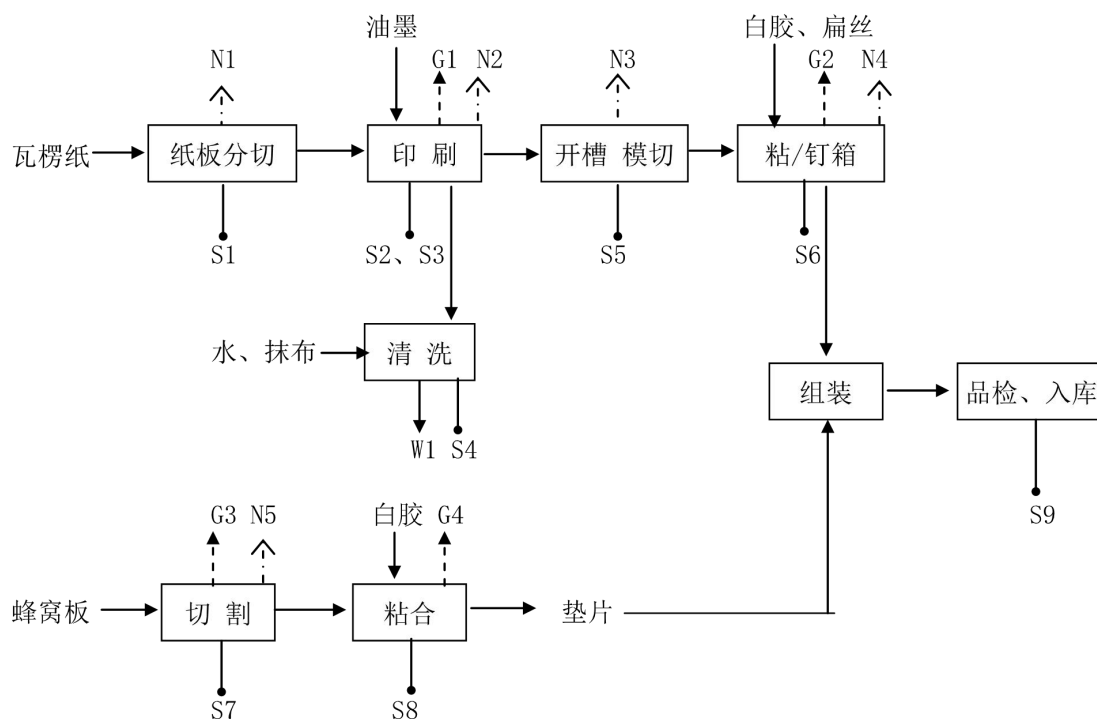
图 2-3 瓦楞纸箱生产工艺流程图
