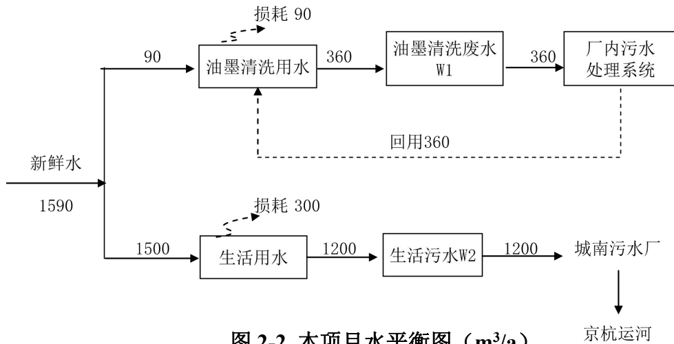
图 2-2 本项目水平衡图 (m³/a)
